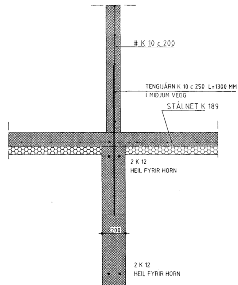
SNID - B 1:20
