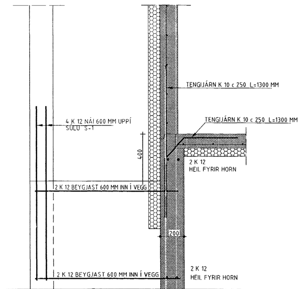
SNID - C 1:20
