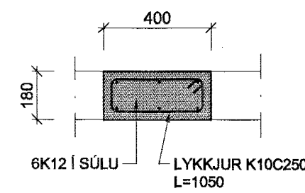
SÚLA S1 1:20
