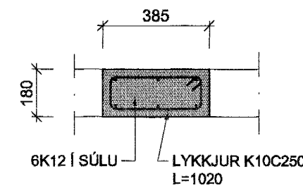
SÚLA S3 1:20
