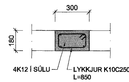
SÚLA S2 1:20
