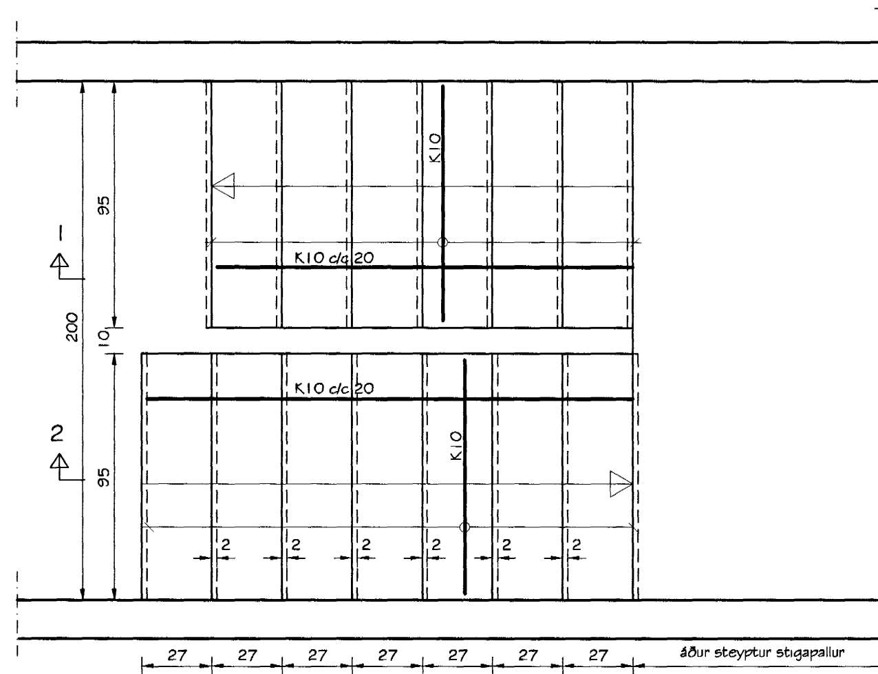
GAUKSÁS 17 - SIGI INNAHÚSS MÁLSETNING OG JÁRNALÖGN - GRUNNMYND MKV. 1:20
