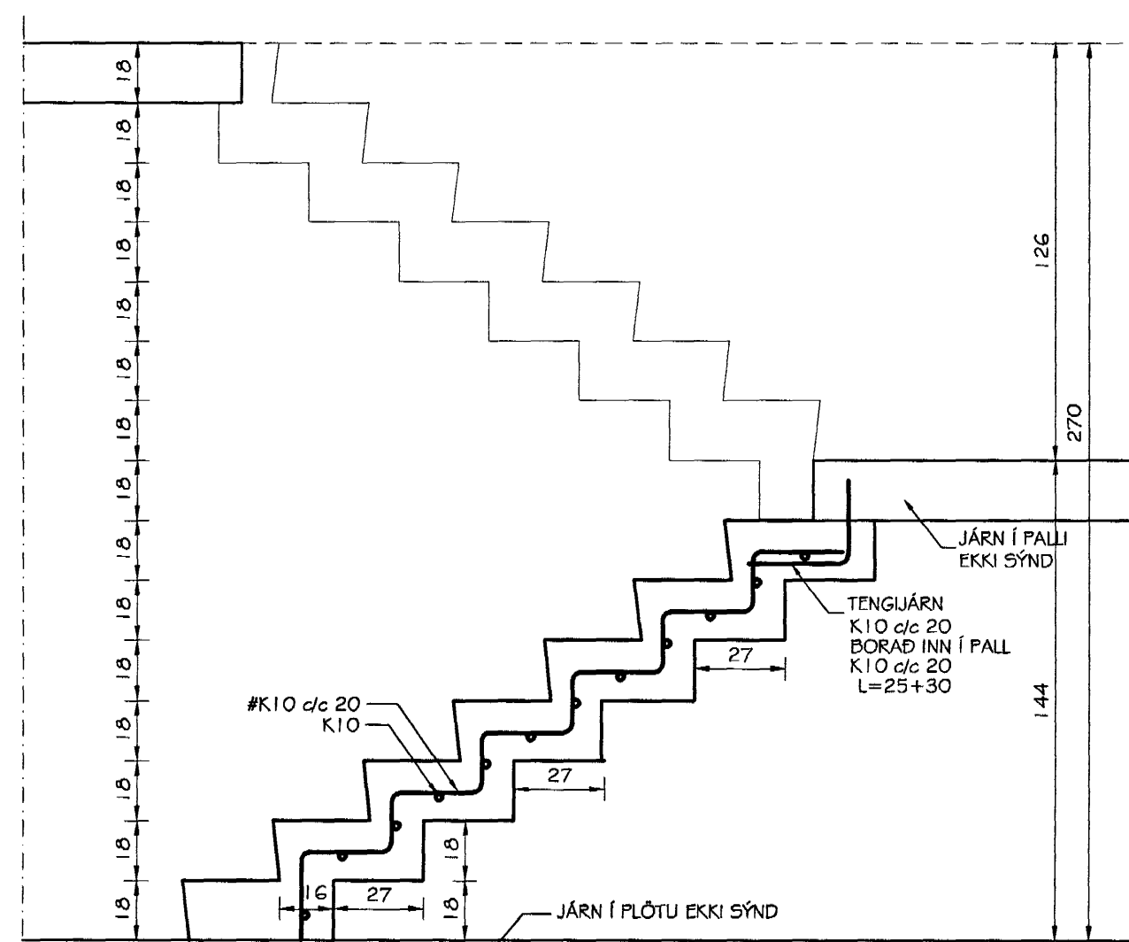
STIGI MÁLSETNING OG JÁRNALÖGN - SNIÐ 2-2 MKV. 1:20
