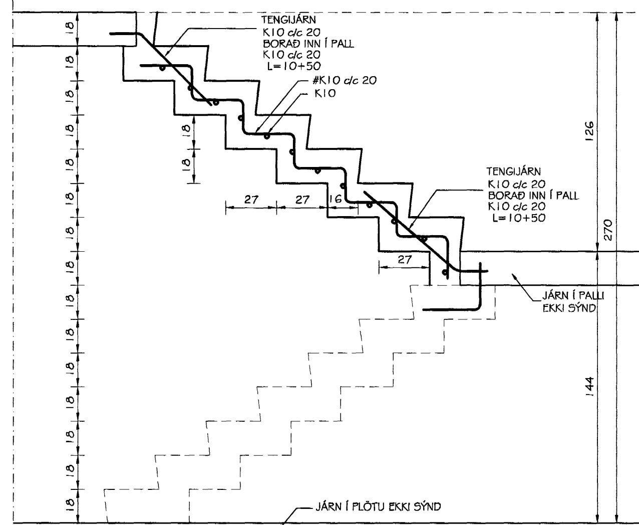
STIGI MÁLSETNING OG JÁRNALÖGN - SNIÐ 1-1 MKV. 1:20
