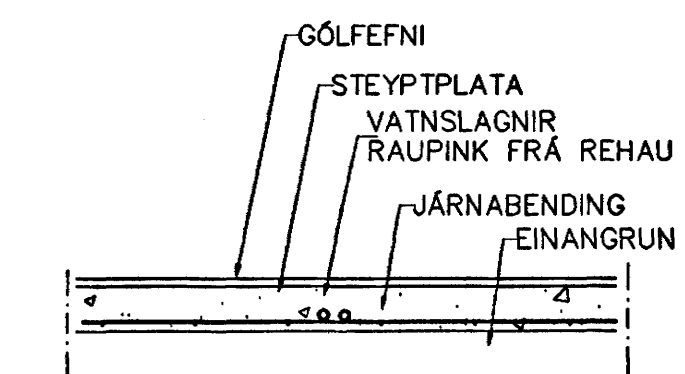
LAGNIR, SNIÐ, 1:20
