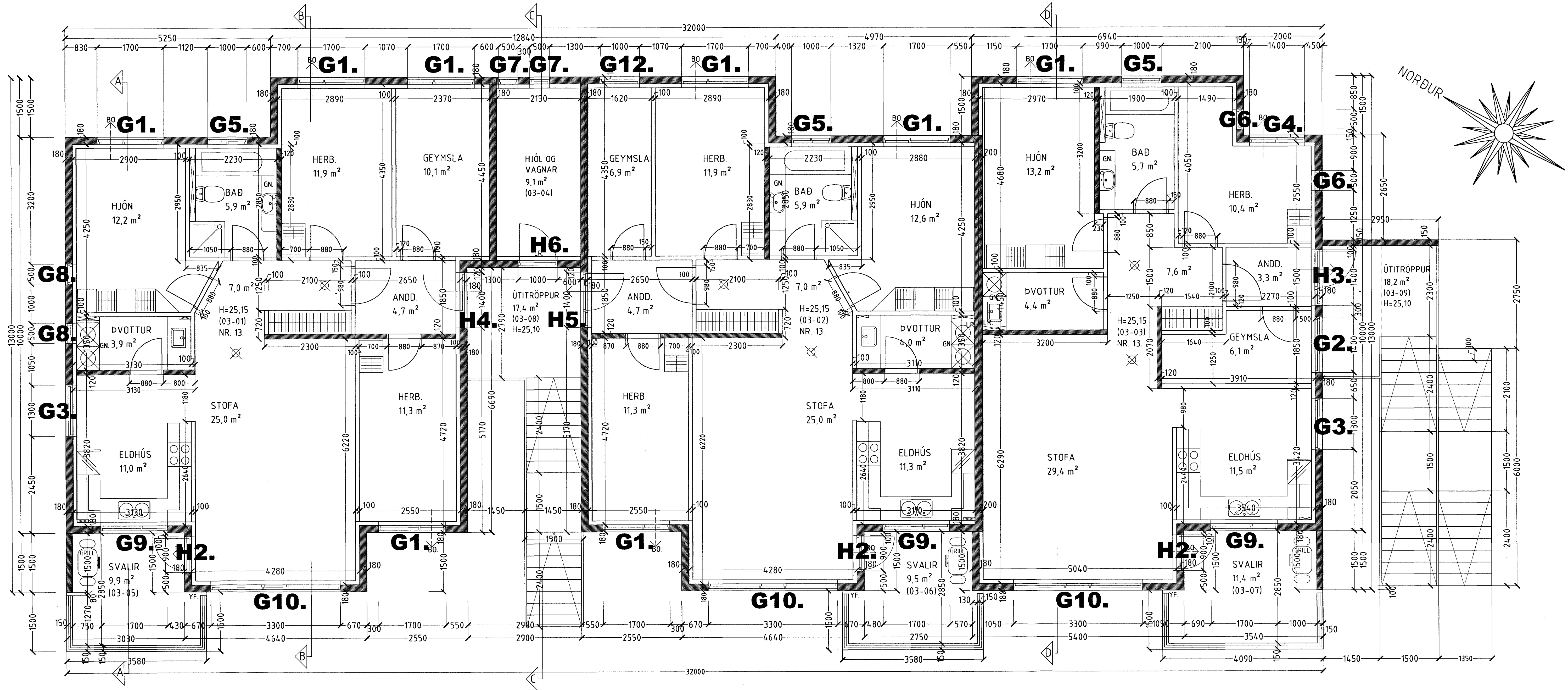
GRUNNMYND 3. HÆÐ MKV. 1:50.
