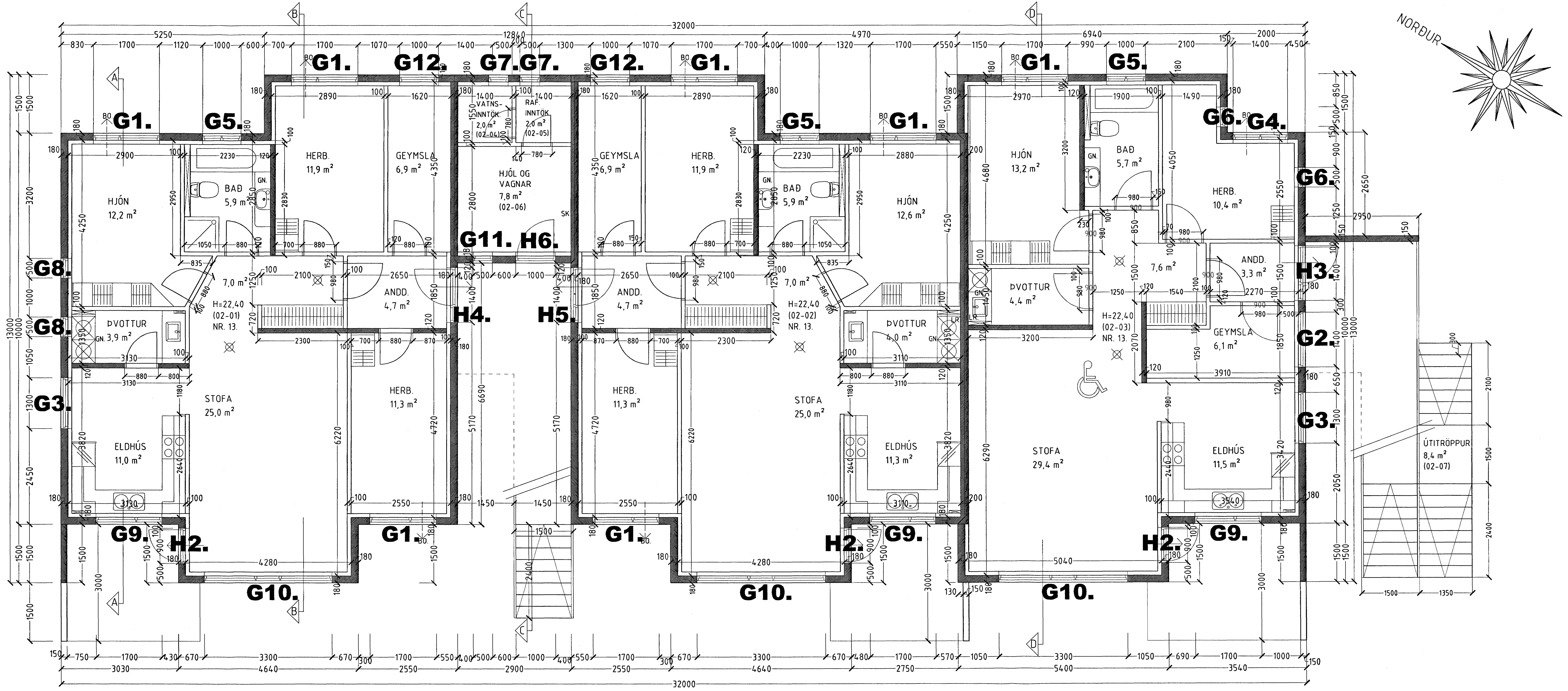
GRUNNMYND 2. HÆÐ MKV. 1:50.
