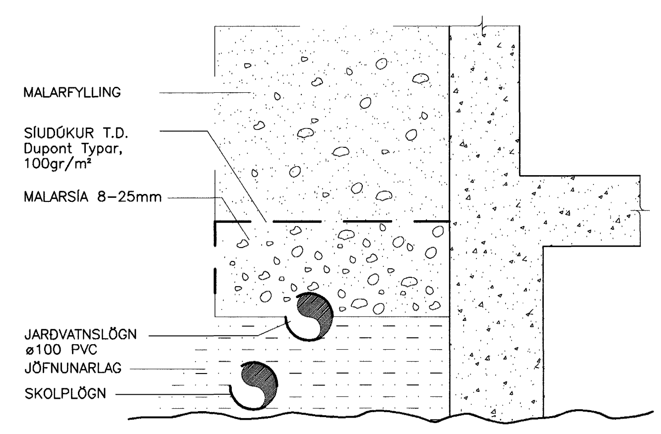
FRÁGANGUR JARÐVATNSLAGNA ÚR PVC 1:10
