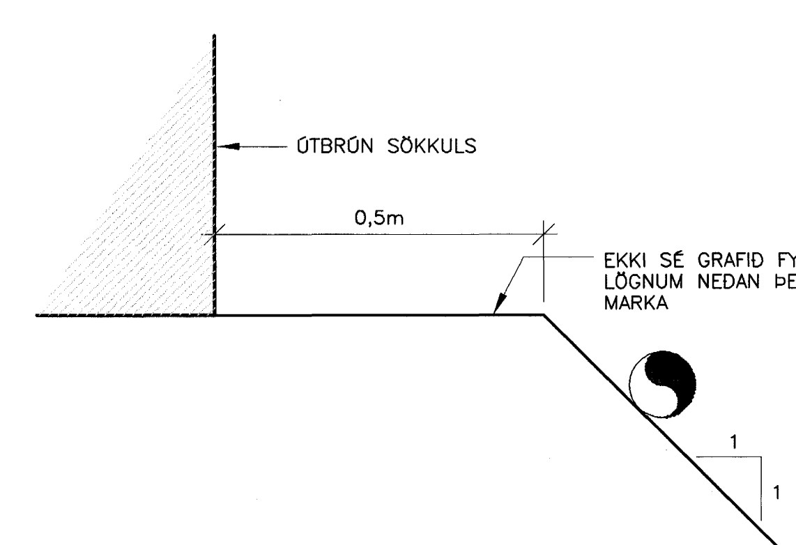
LEGA LAGNA VID HÚS 1:10
