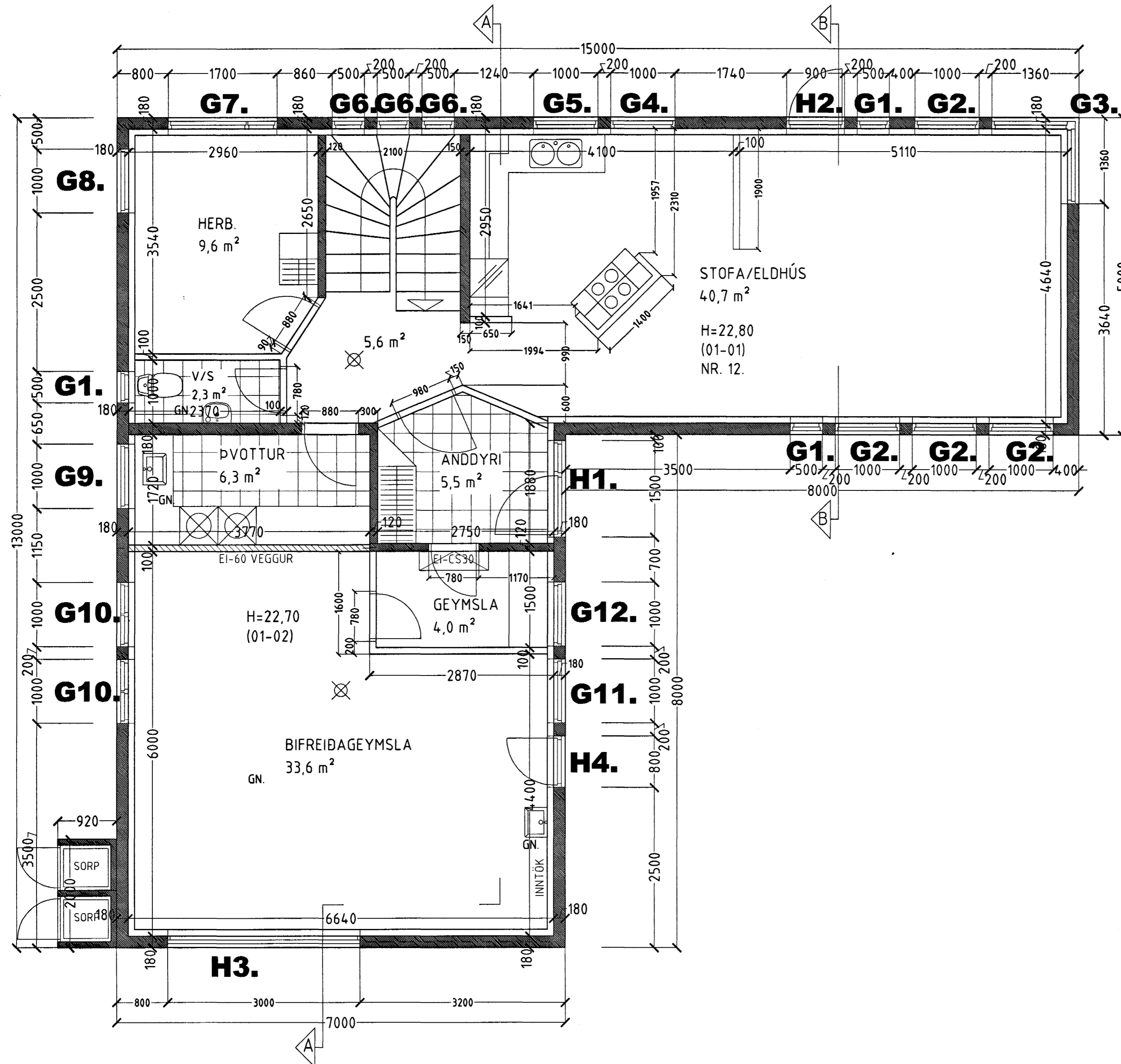
GRUNNMYND 1 HÆÐ MKV. 1:50.
