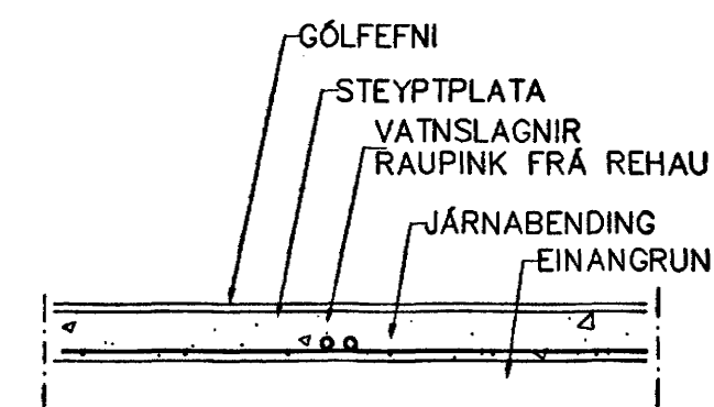
LAGNIR, SNIÐ, 1:20
