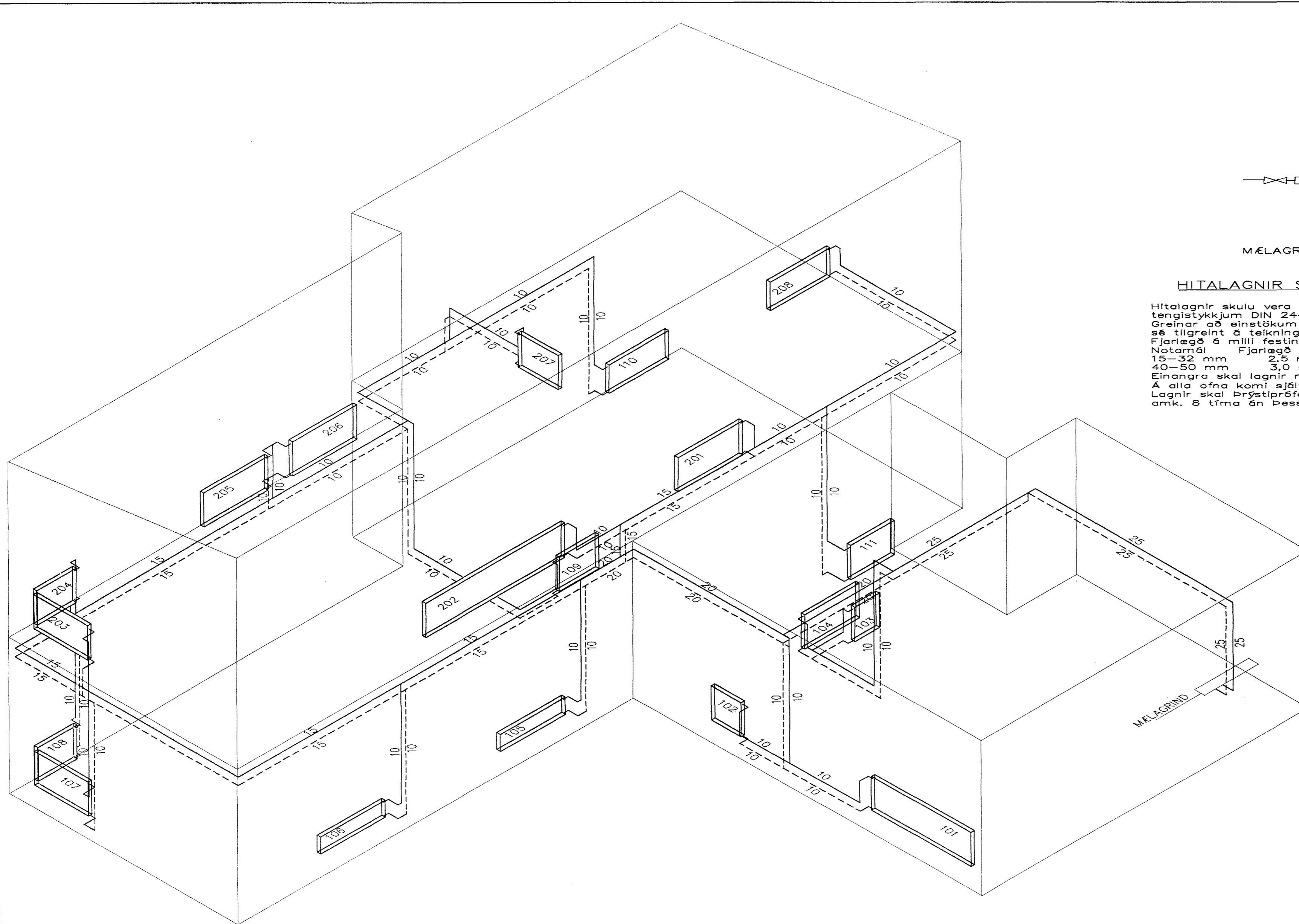
RÚMMYND HITALAGNA 1:50
