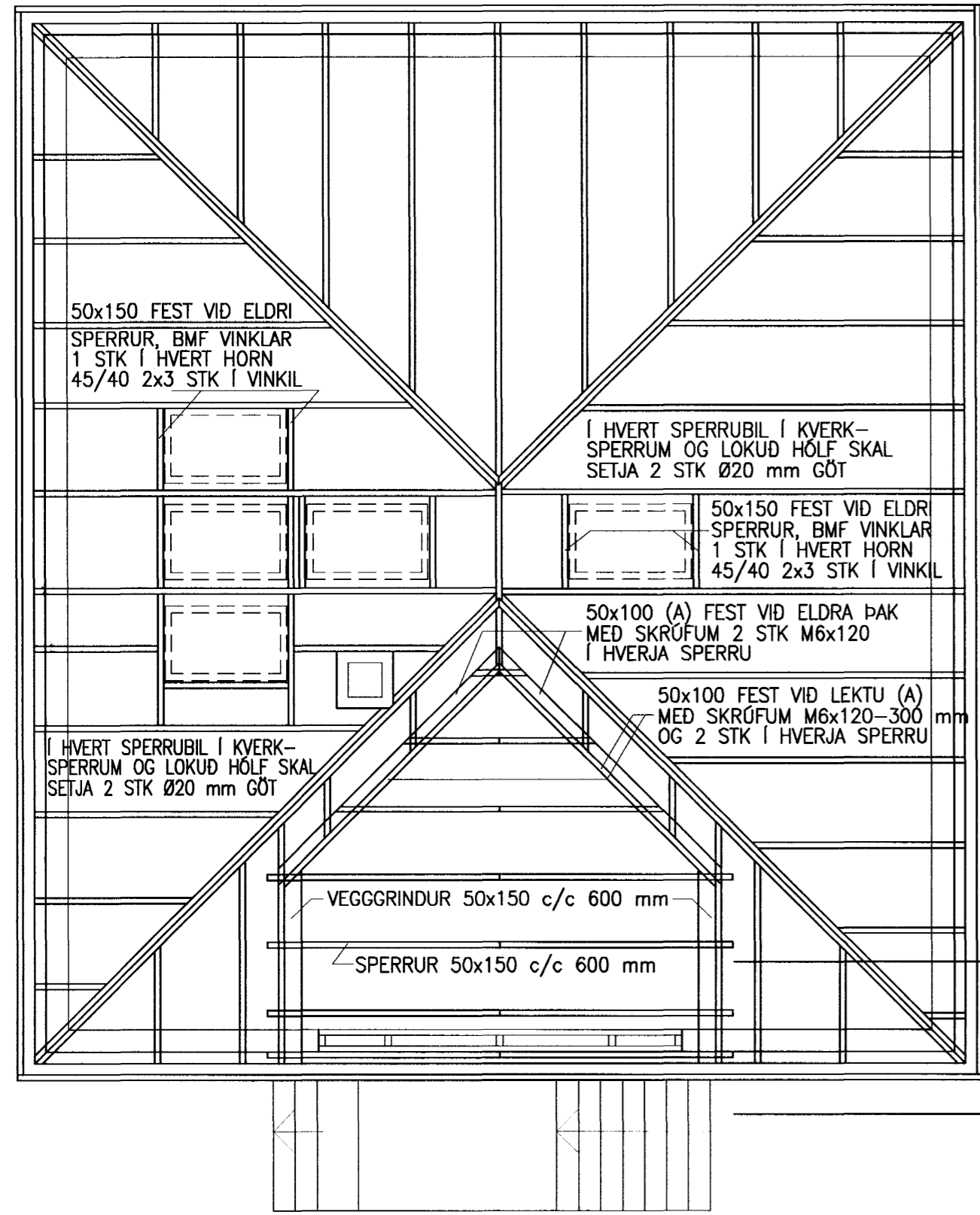
SPERRUPLAN 1:50
