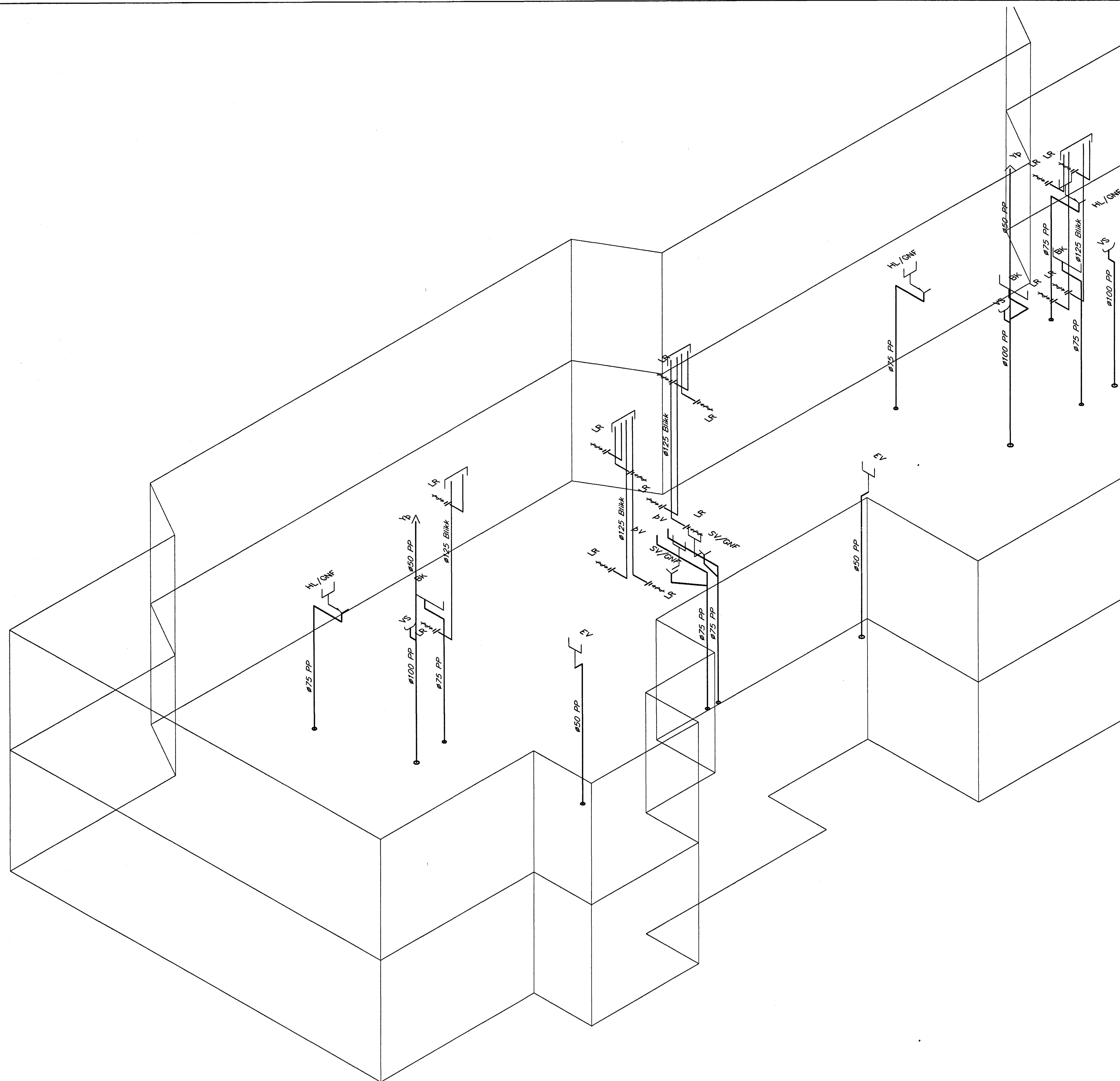
Fráveitulagnirlagnir, Rúmmynd, 1:50
