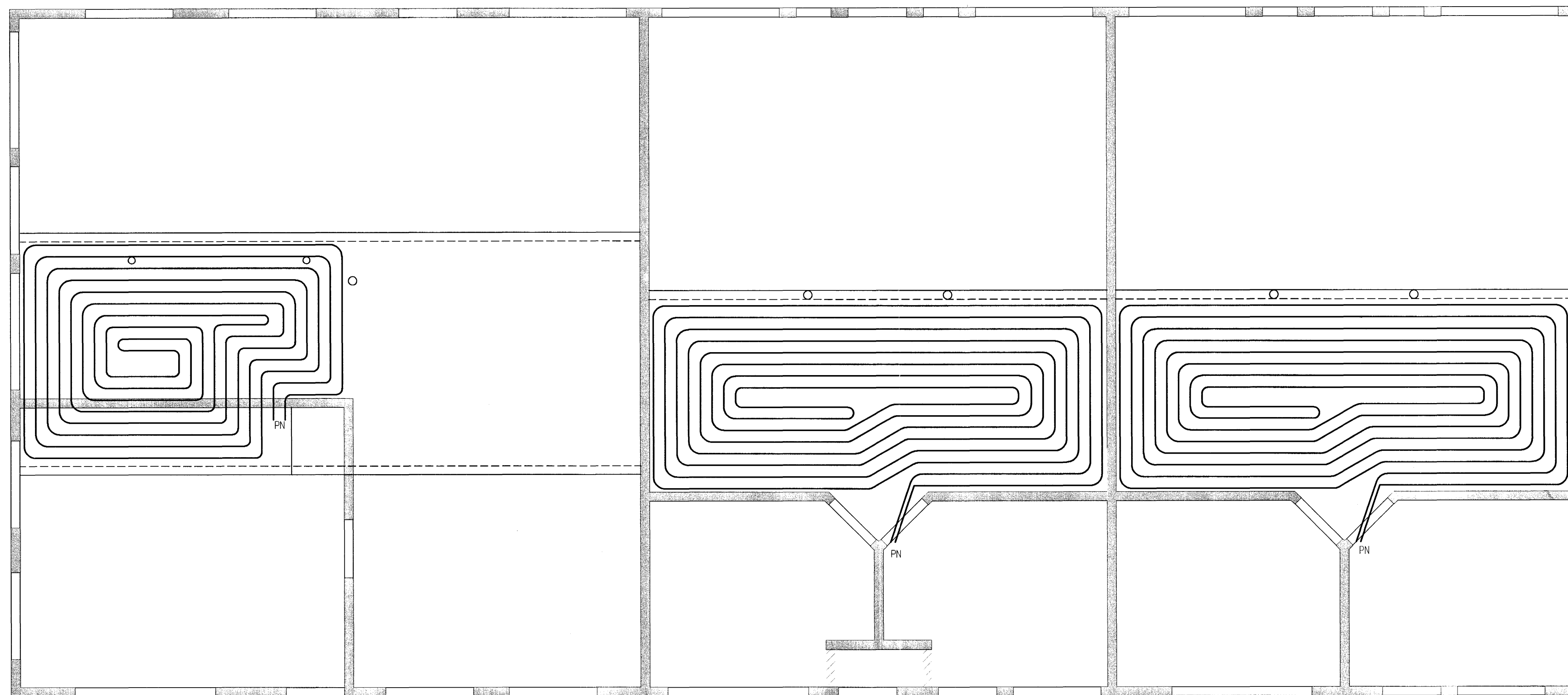
GÓLFHITALAGNIR GRUNNMYND EFRÍ HÆÐAR
