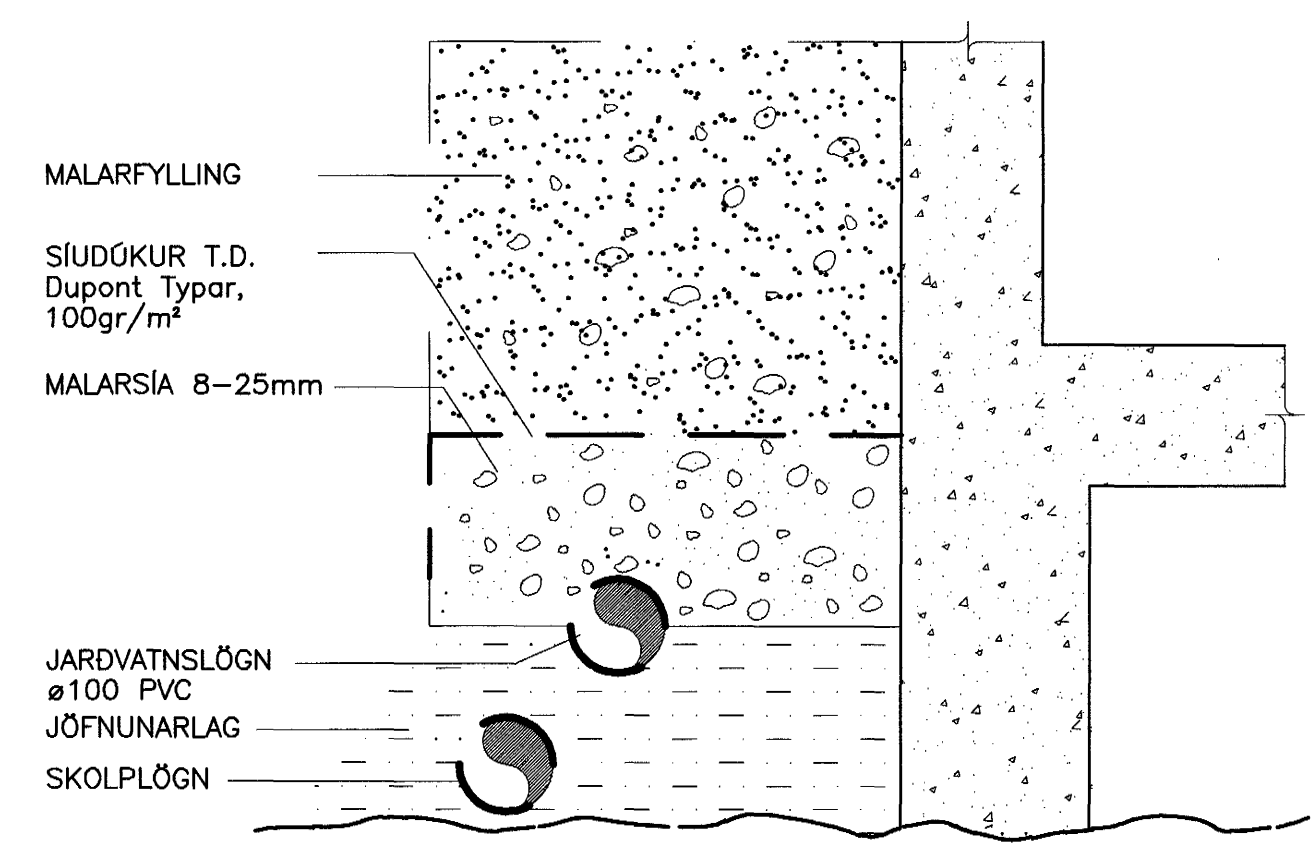
FRÁGANGUR JARÐVATNSLAGNA ÓR PVC 1:10
