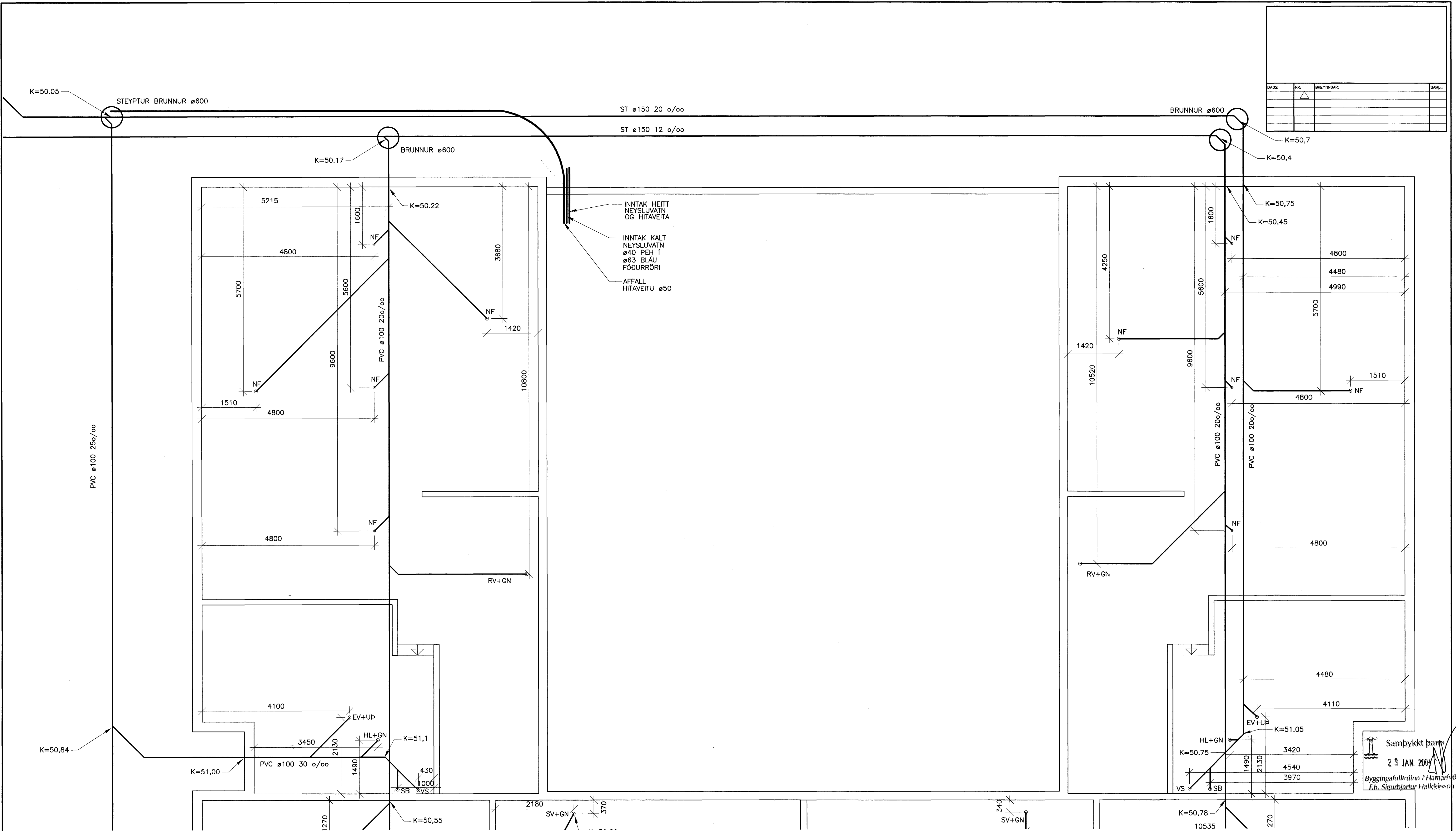
GRUNNLAGNIR GRUNNMYND. 1:50
