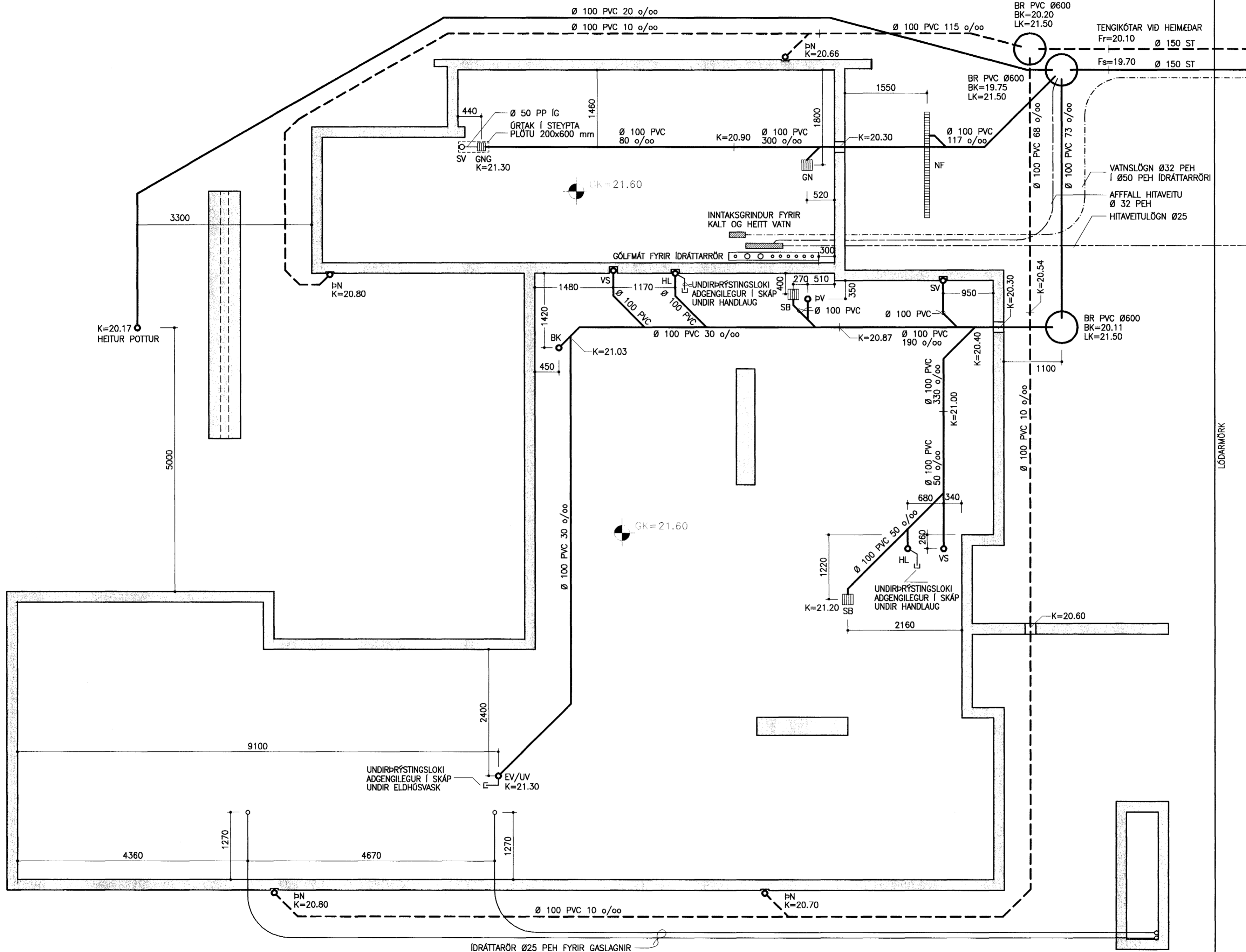
GRUNNMYND FRÆRENNISLAGNIR 1:50
