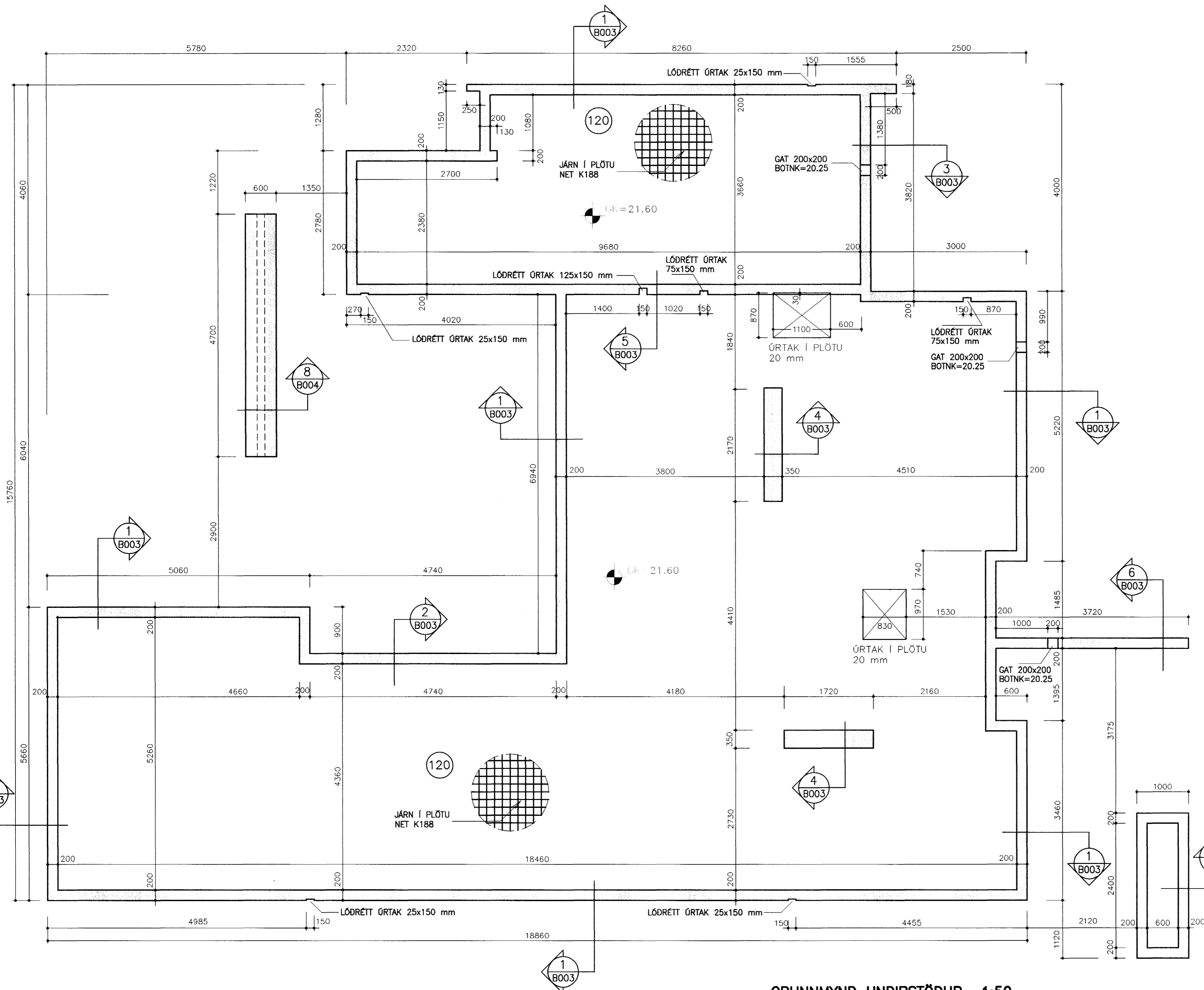
GRUNNMYND UNDIRSTÖÐUR 1:50
