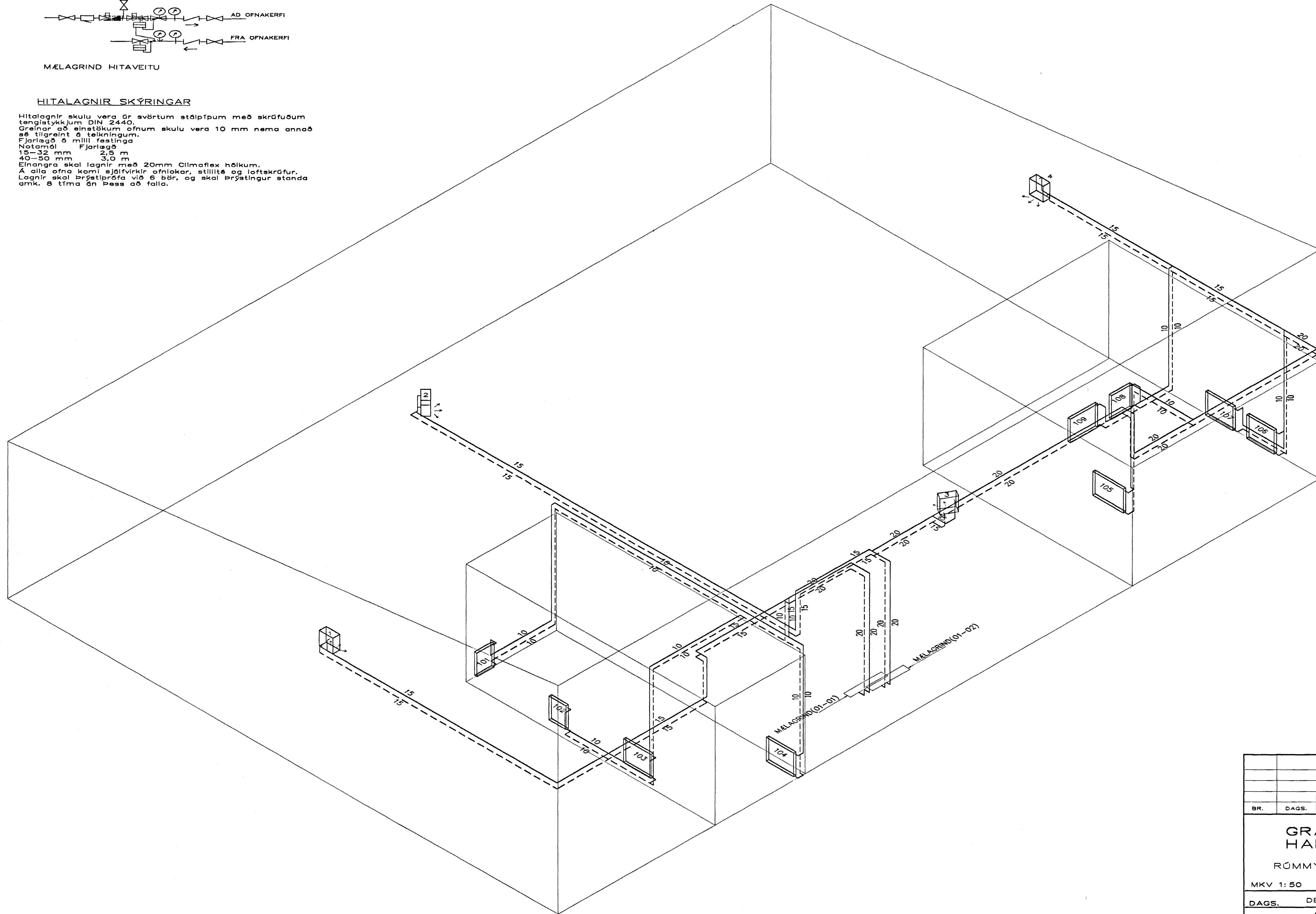
RÚMMYND HITALAGNA 1:50
