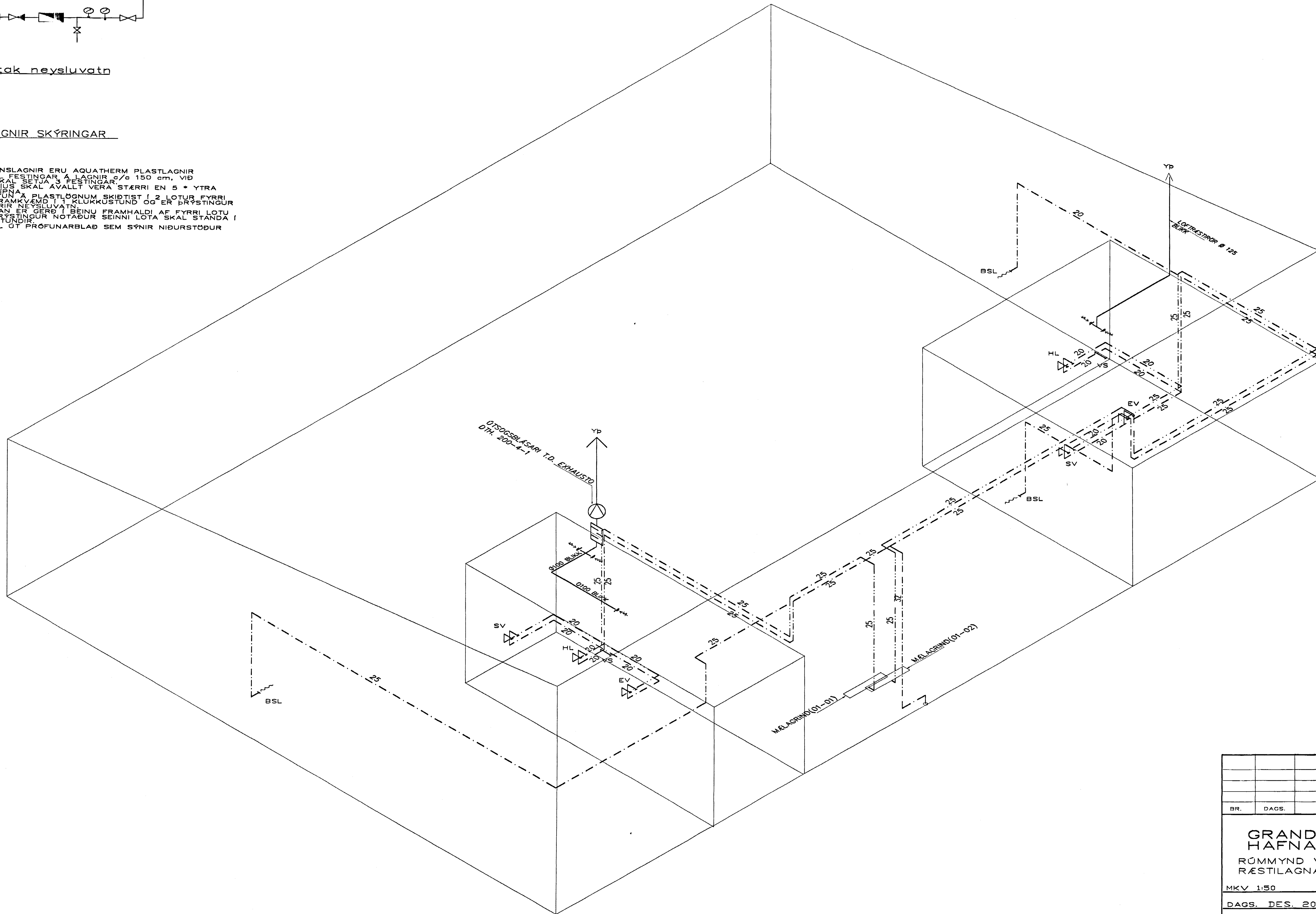
RÚMMYND VATNS OG LOFTRÆSTILAGNA 1:50
