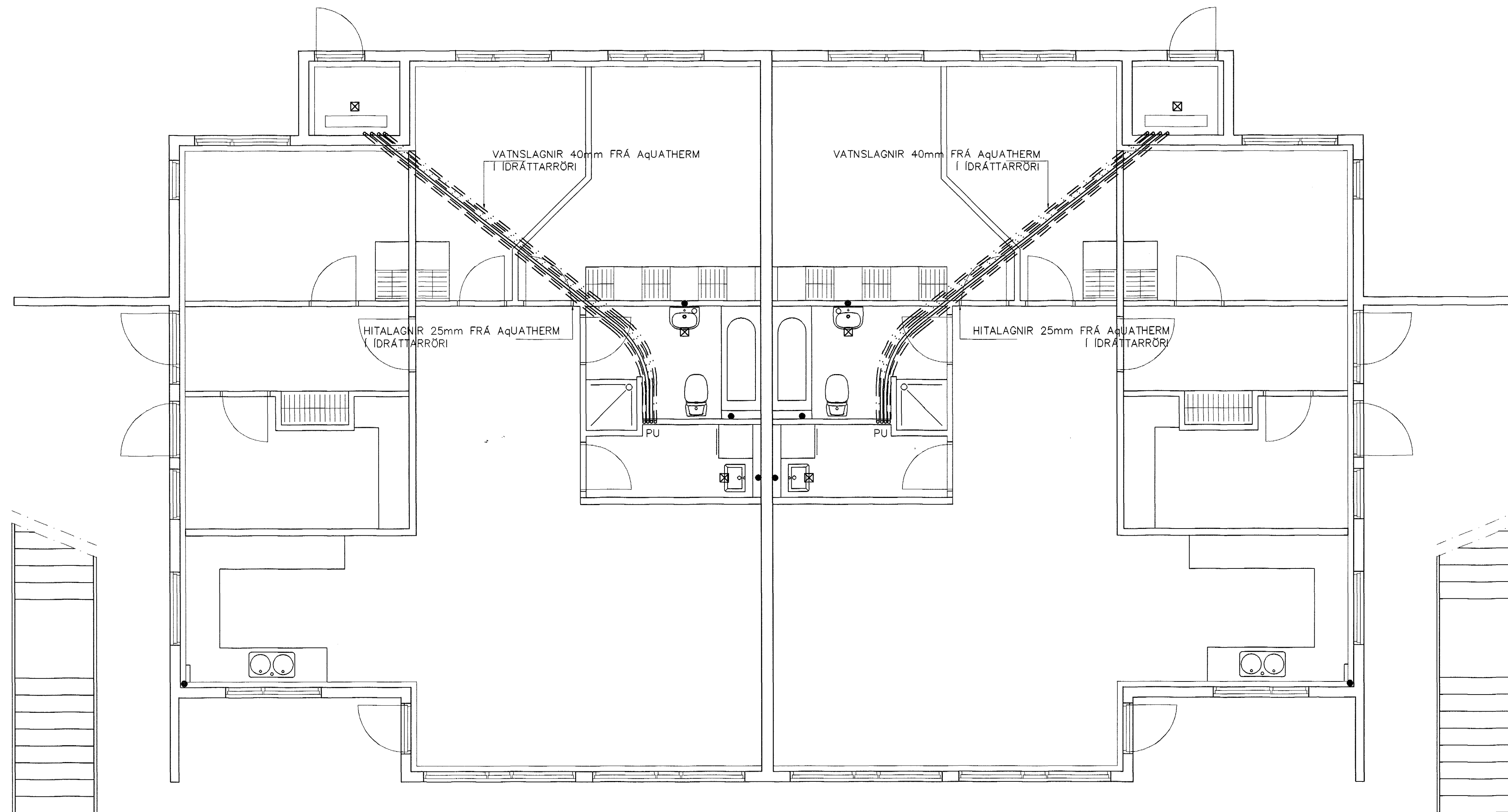
GRUNNMYND 1:50
