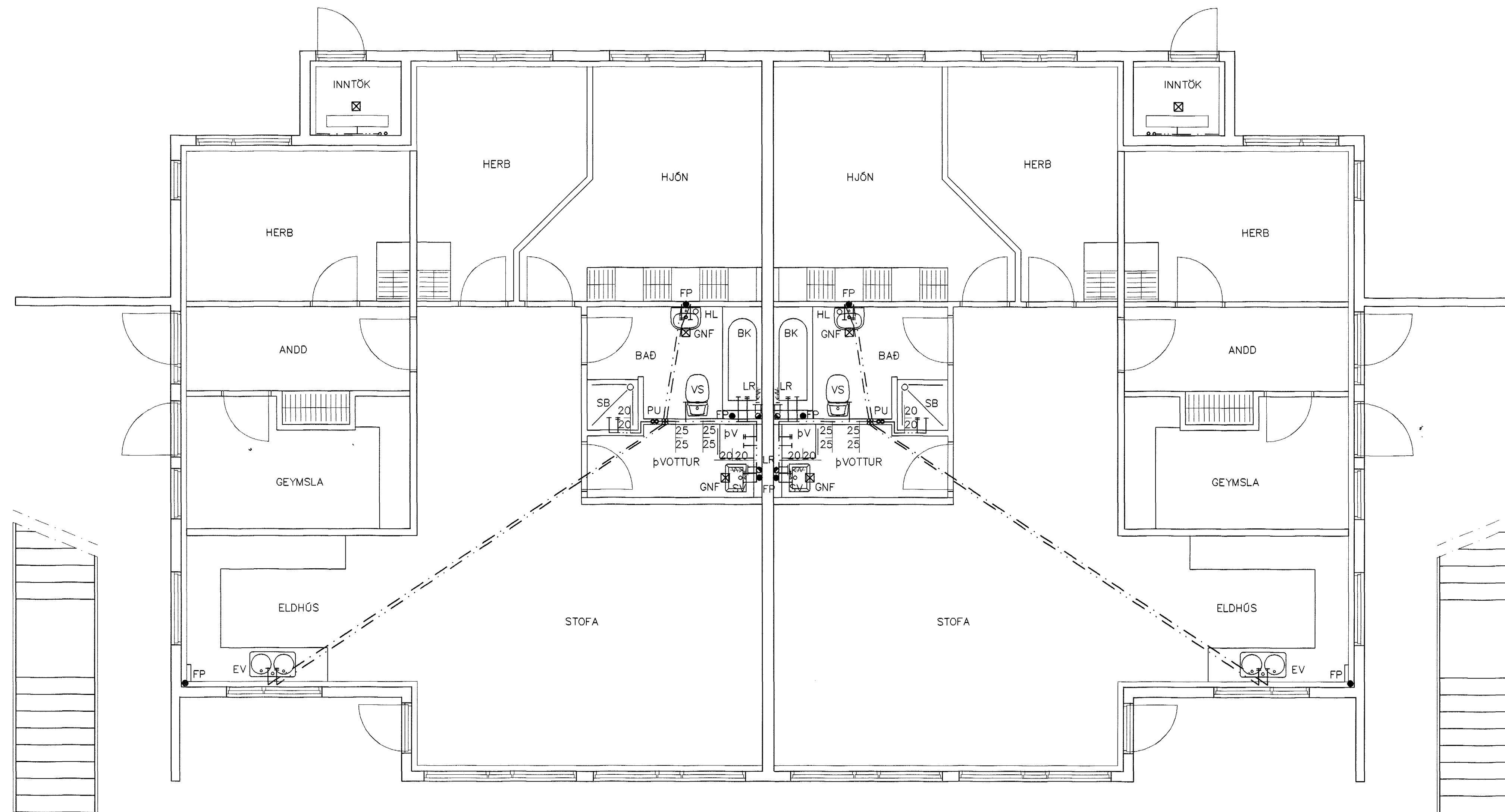
GRUNNMYND 1 HÆÐAR 1:50
