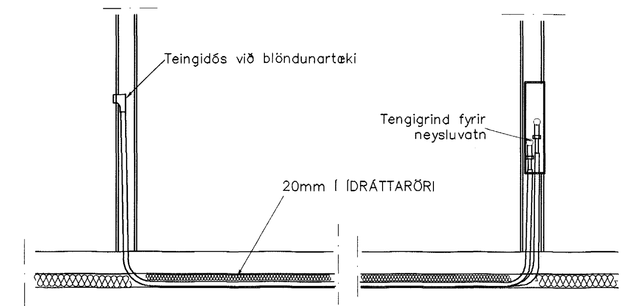
TENING NEYSLUVATNSLAGNA 1:20
