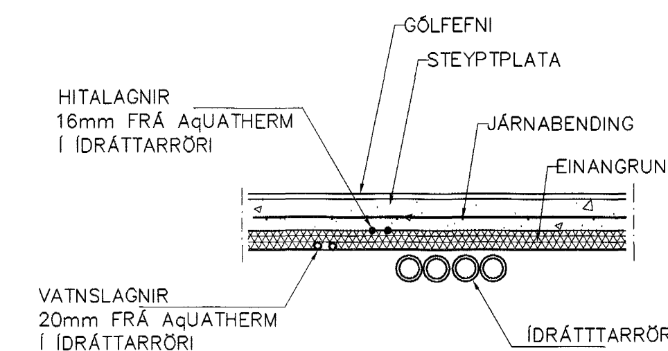
LAGNIR, SNIÐ, 1:20
