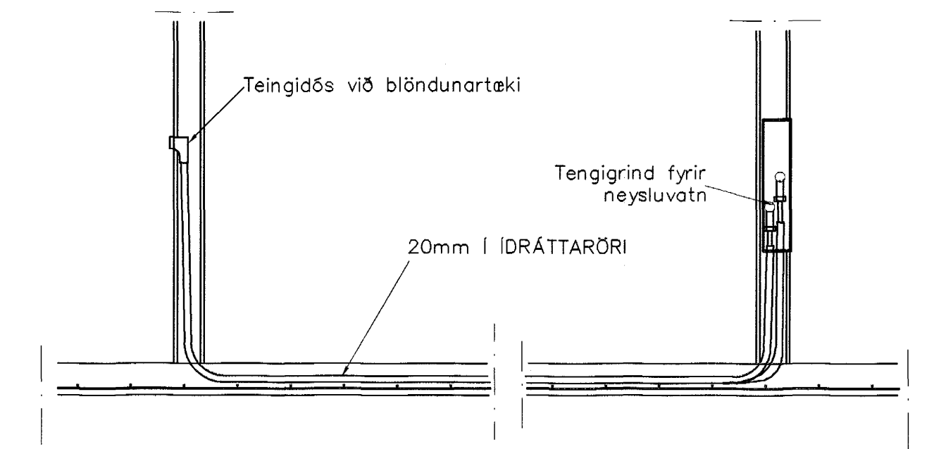
TENING NEYSLUVATNSLAGNA 1:20
