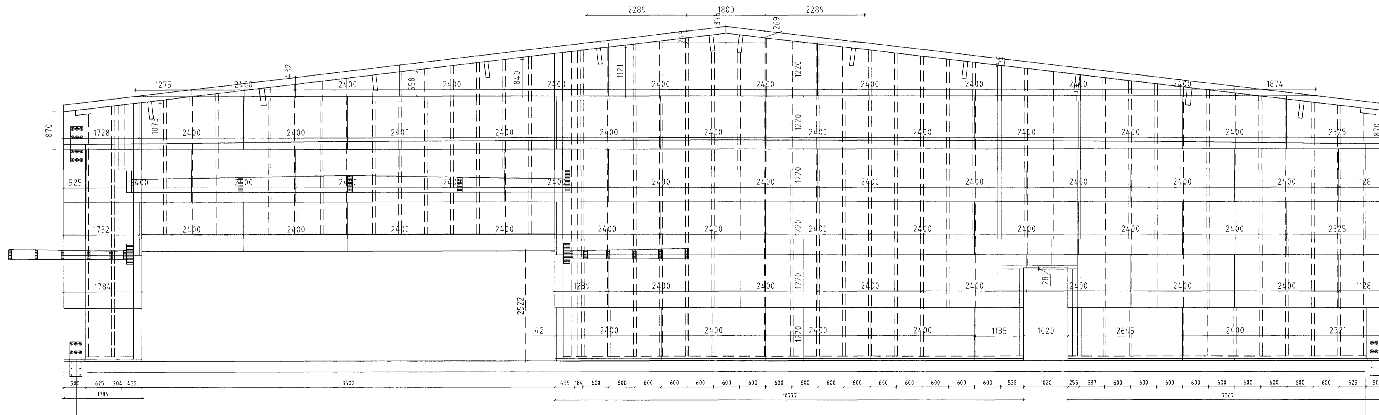
Suðurgafi - krossviðsklæðning úti
