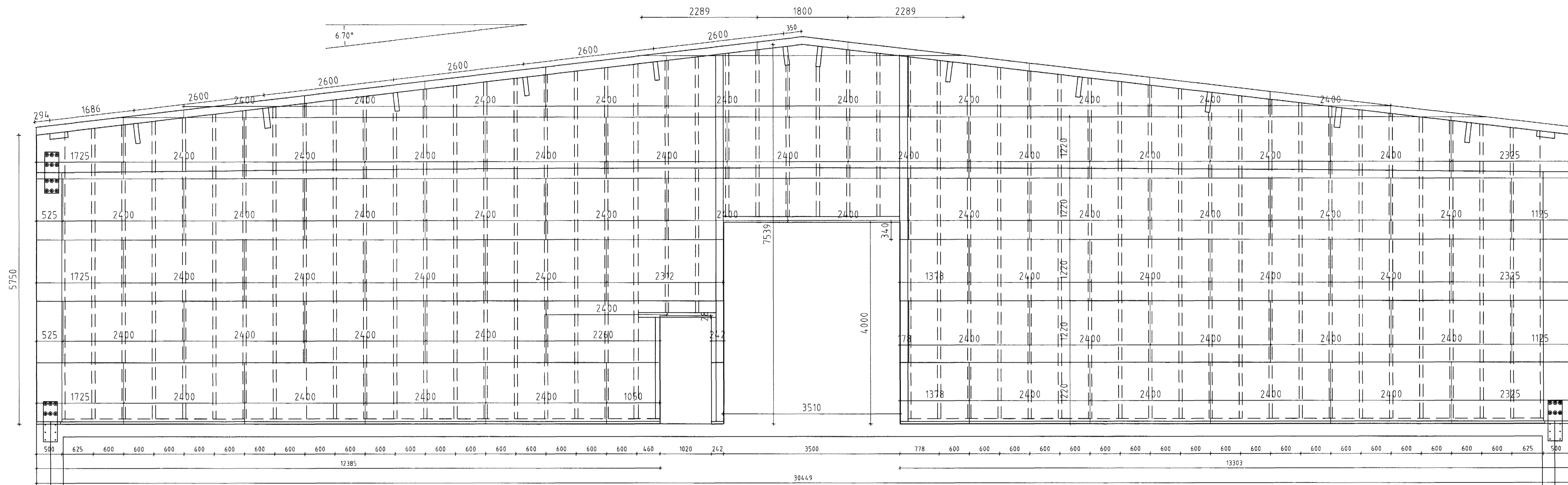
Norðurgafi - krossviðsklæðning úti
