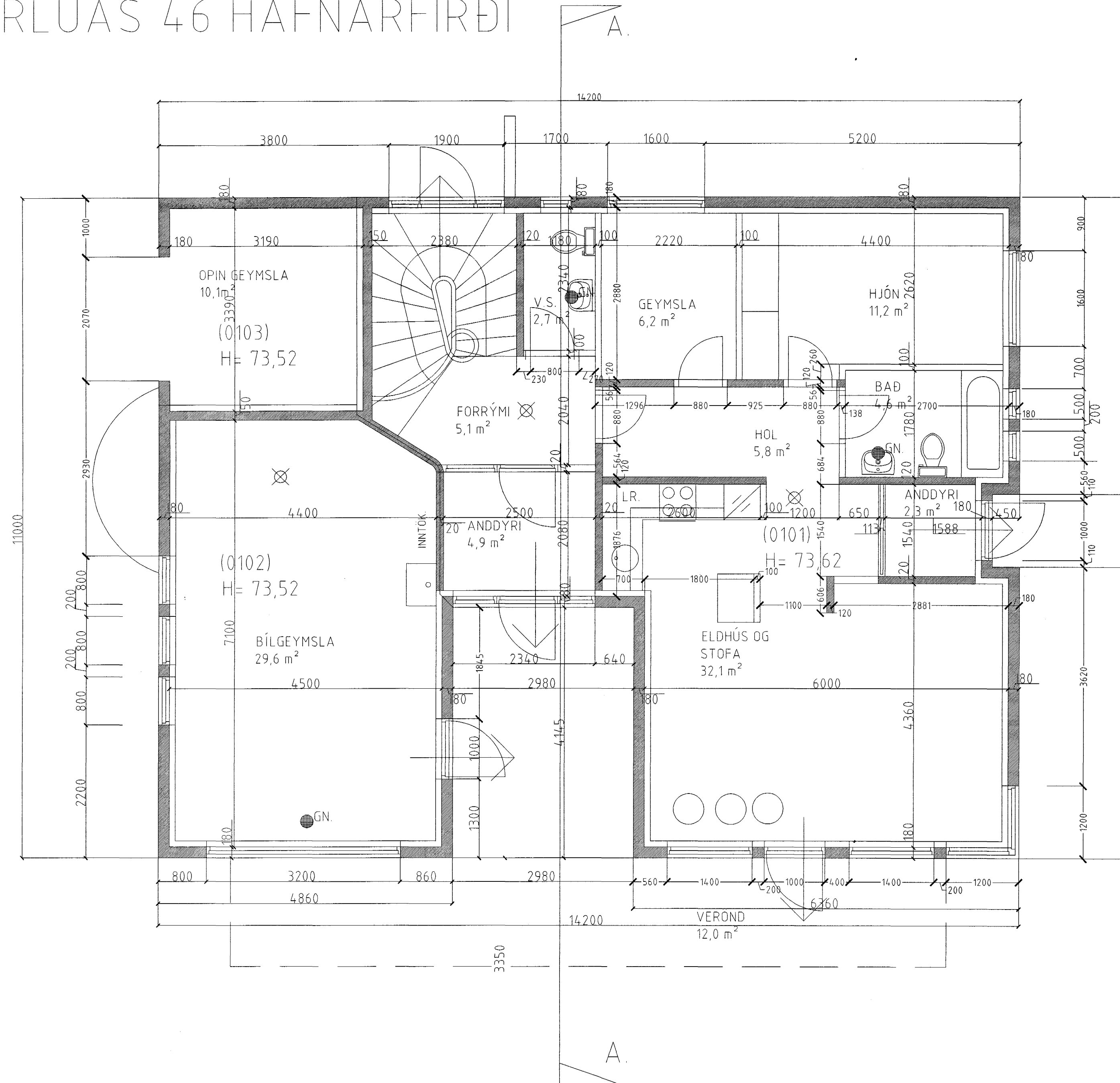
GRUNNMYND 1. HÆÐAR. MKV. 1:50.
