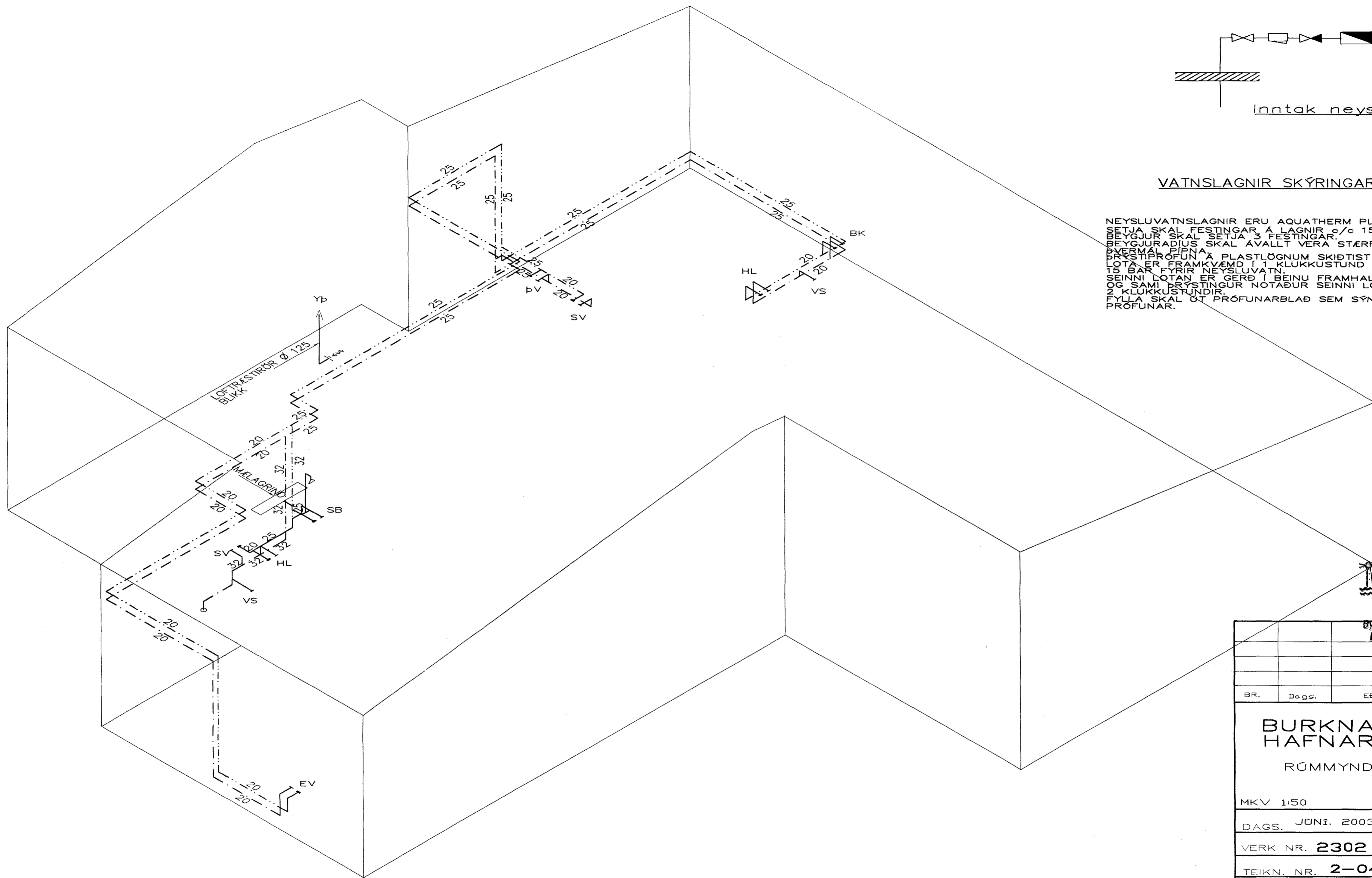
RÚMMYND VATNSLAGNA 1:50
