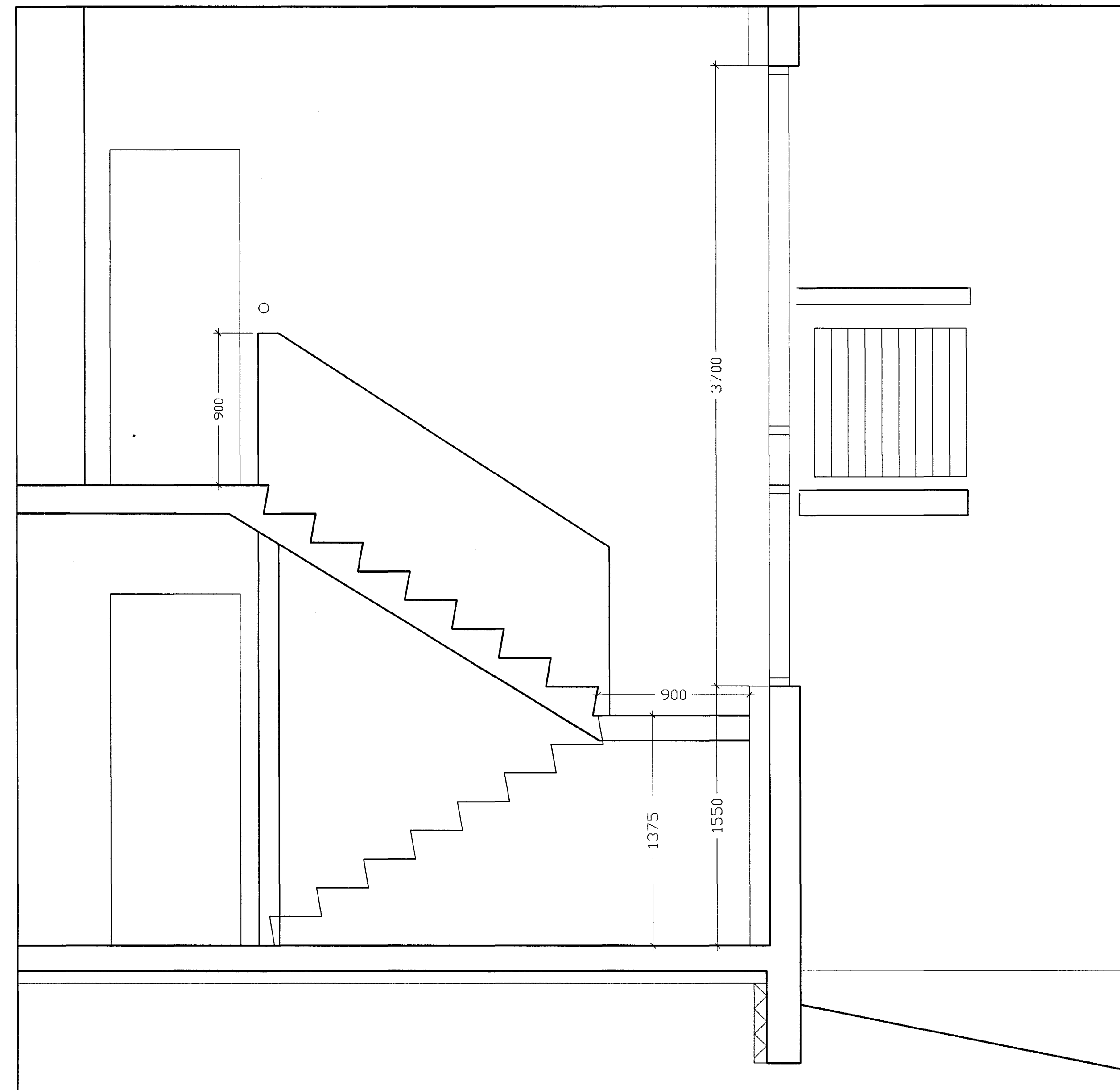
skurður e-e
