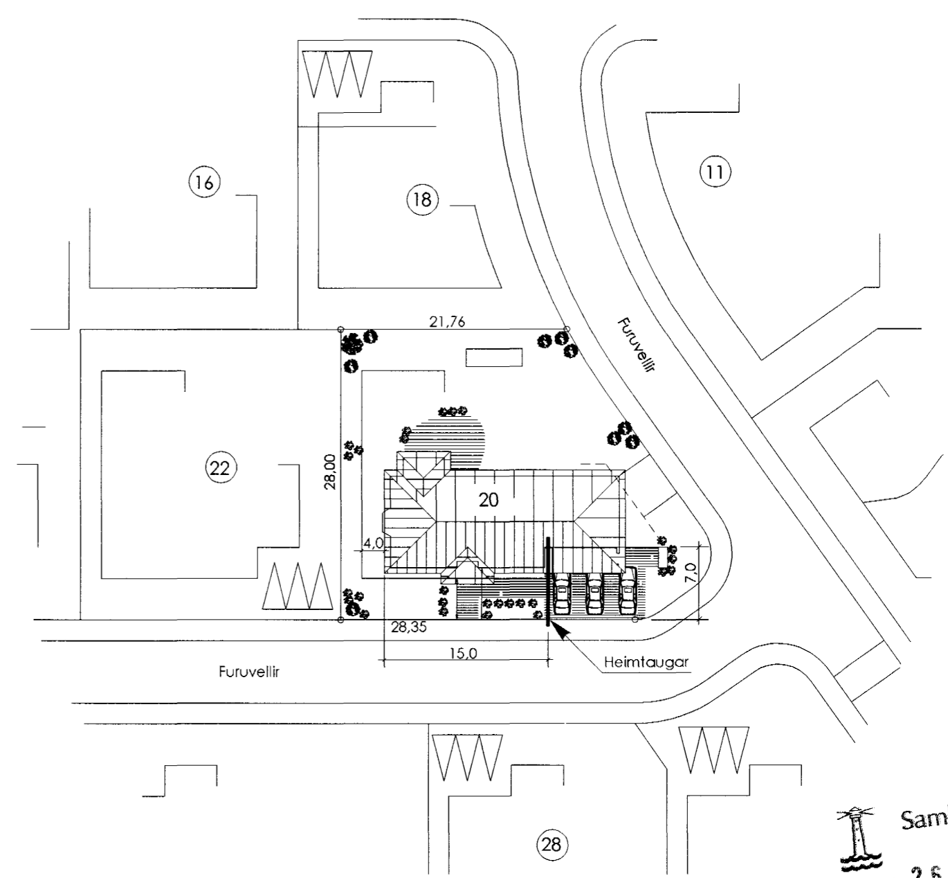
Afstöðunmynd 1:500
