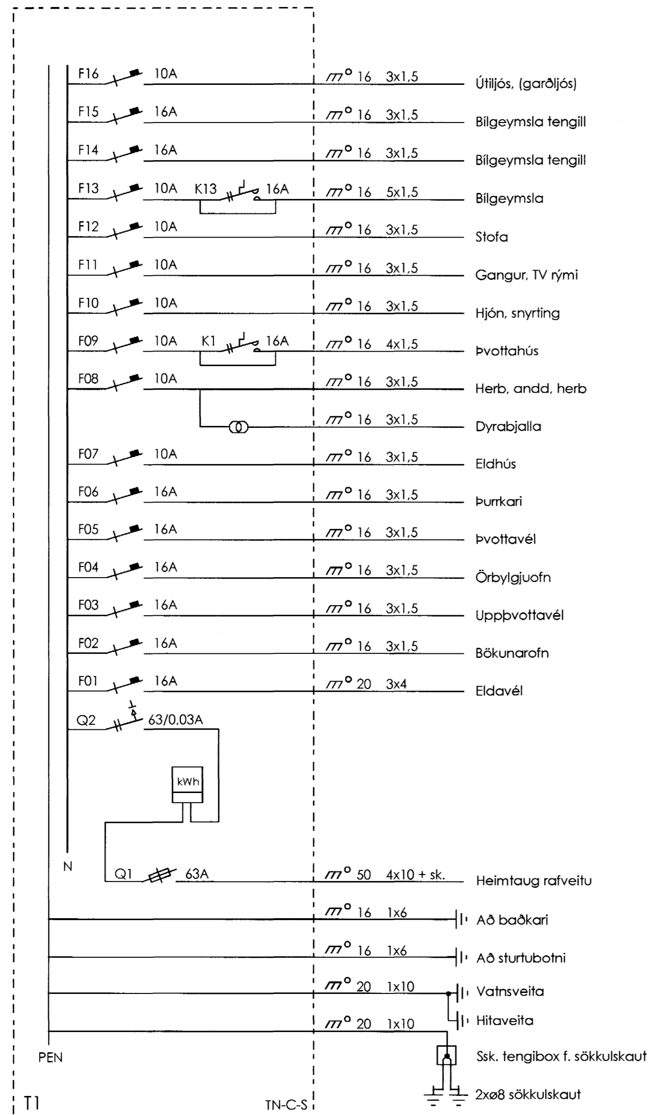
Einlínunmynd
