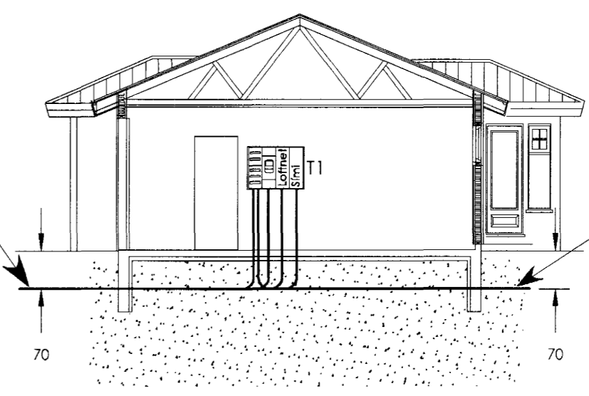
Snið 1:100
