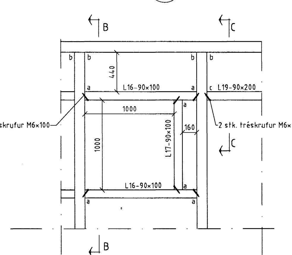
Sérmynd 17 Mkv.: 1:25
