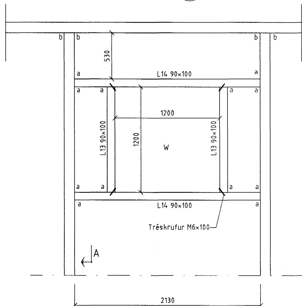
Sérmynd 16 Mkv.: 1:25
