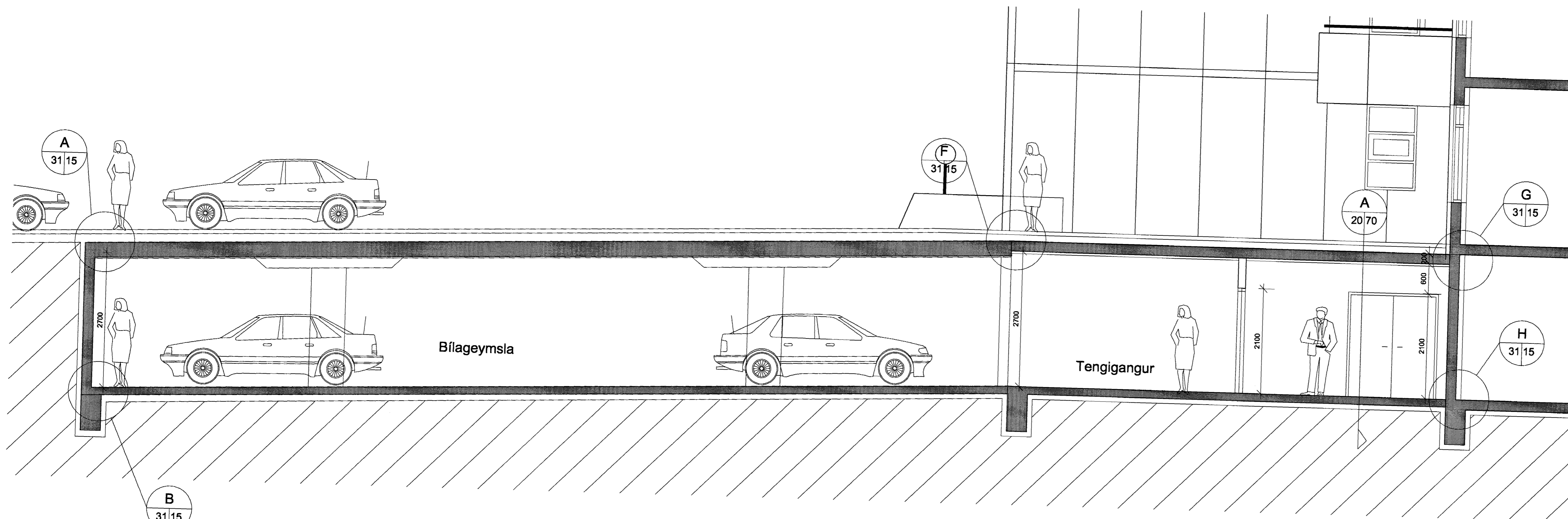
Bílageymsla og tengingangur að Hrafnistu Sneiðing B 1:50
