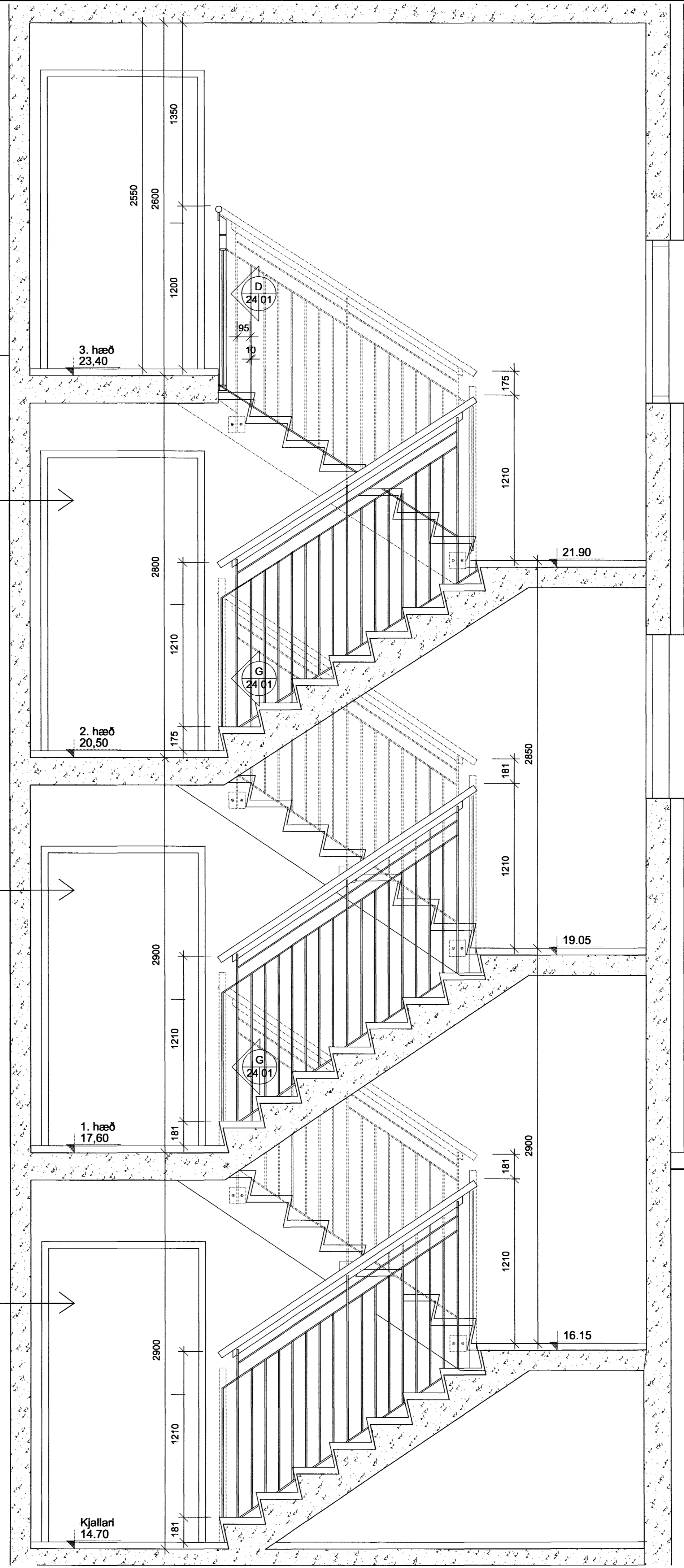
STIGAHÚS HÚSI 2 Sneiðing A - A 1:20
