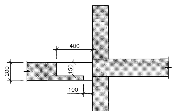
A SNID 1:20 712 712
