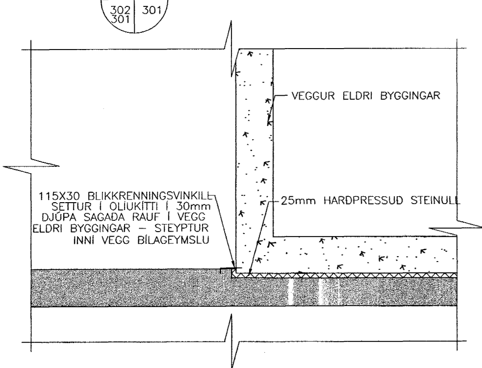
SM8 SÉRMYND 1:20
