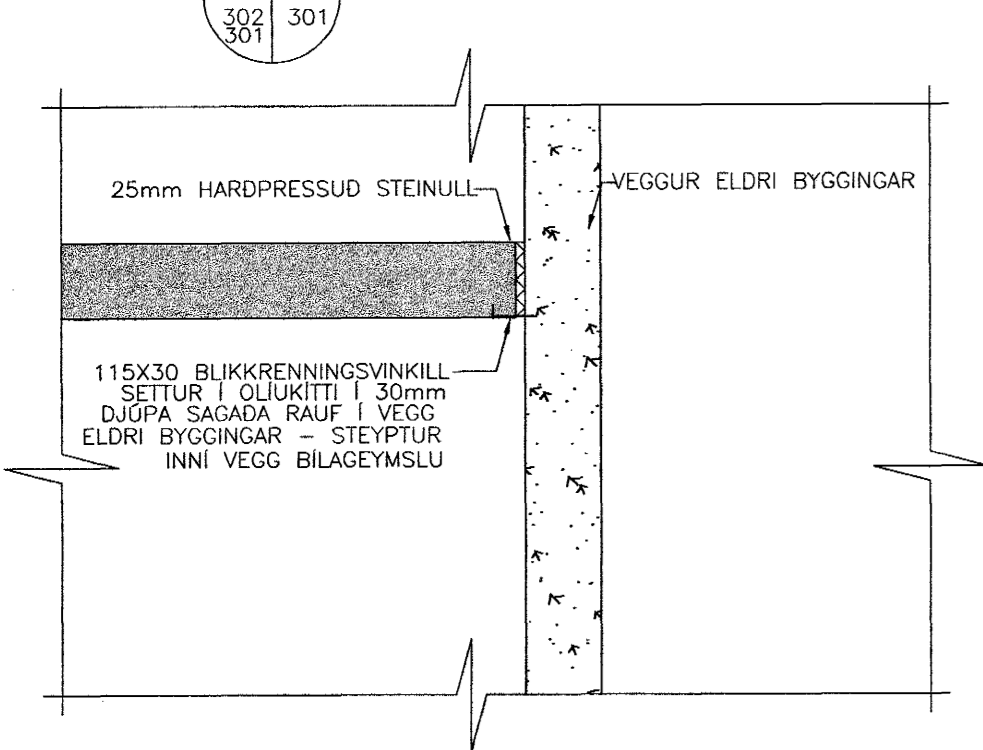
SM7 SÉRMYND 1:20
