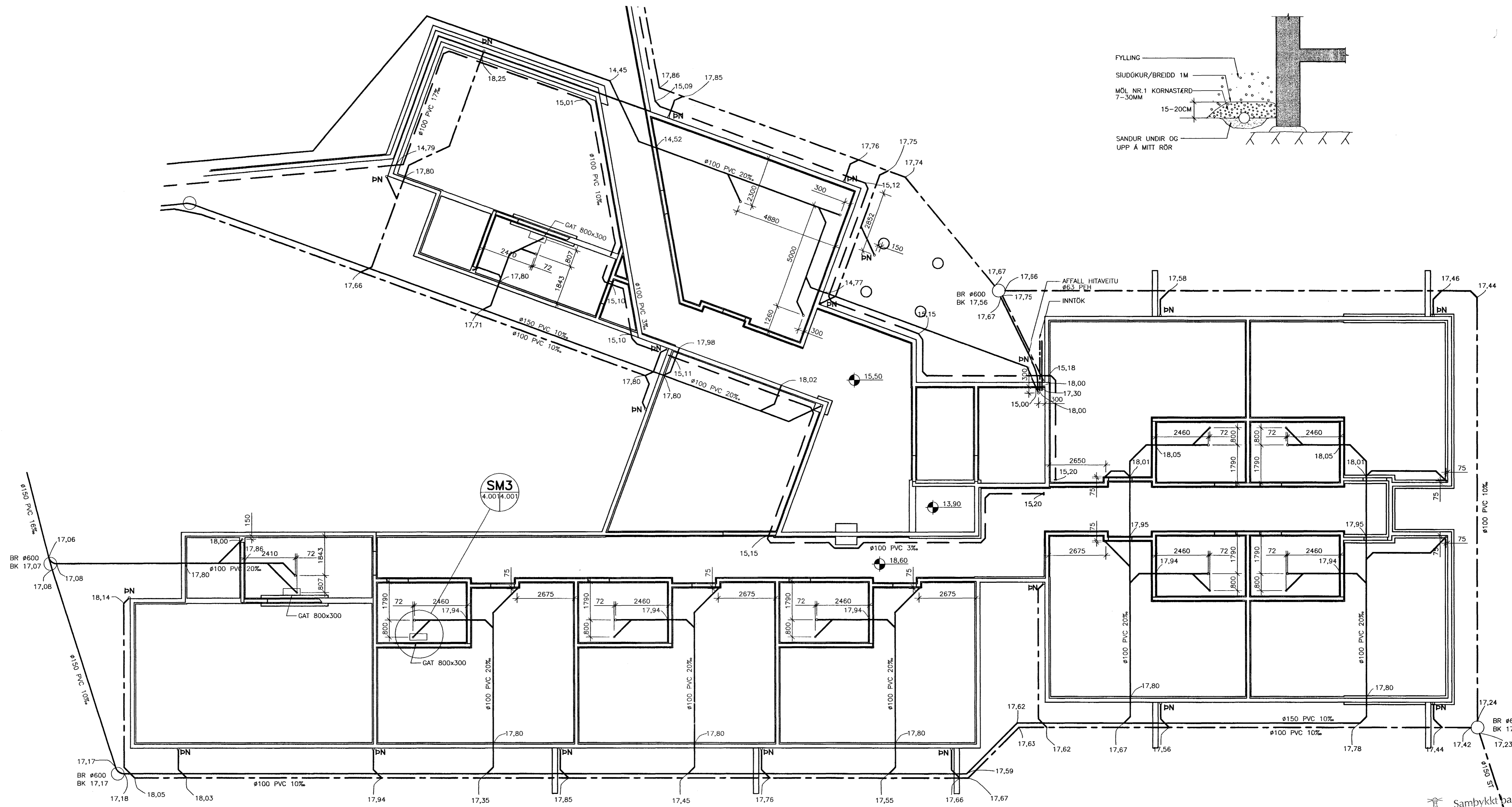
LYKILMYND 1:1000
