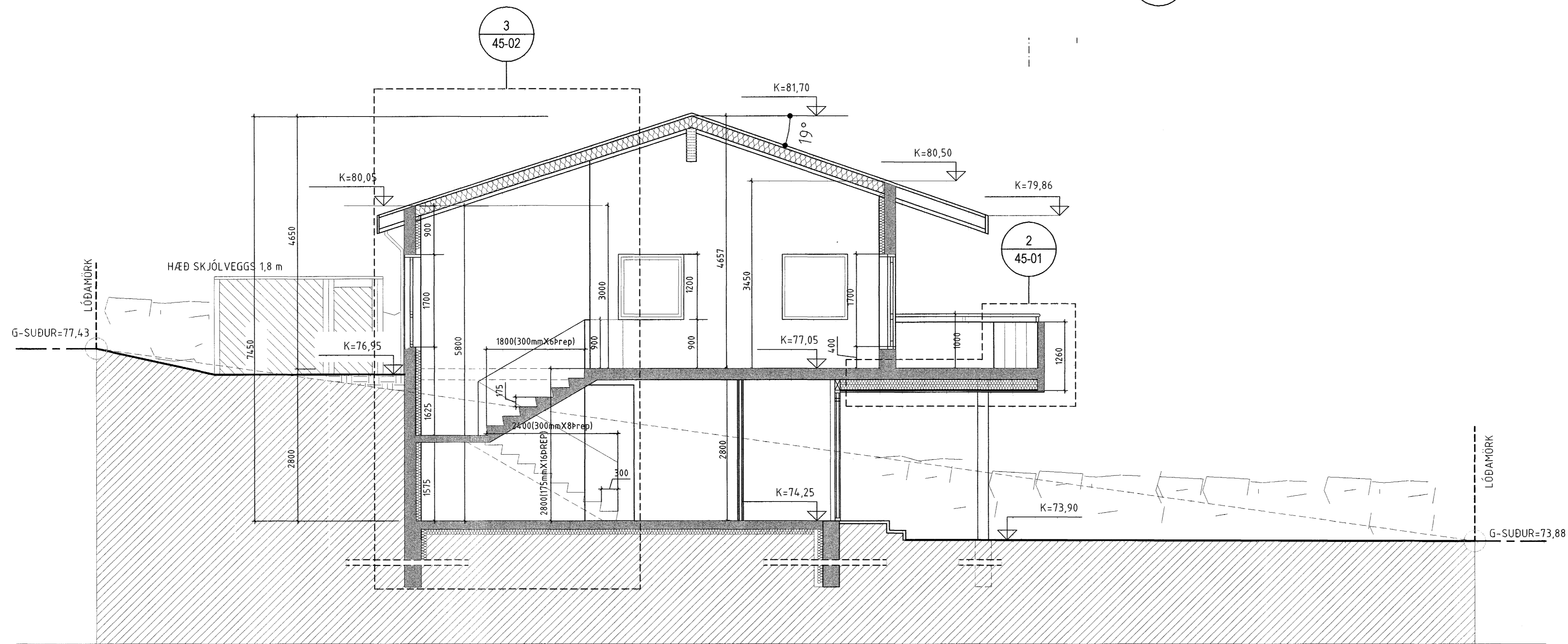
SNEIÐING A-A 1:50
