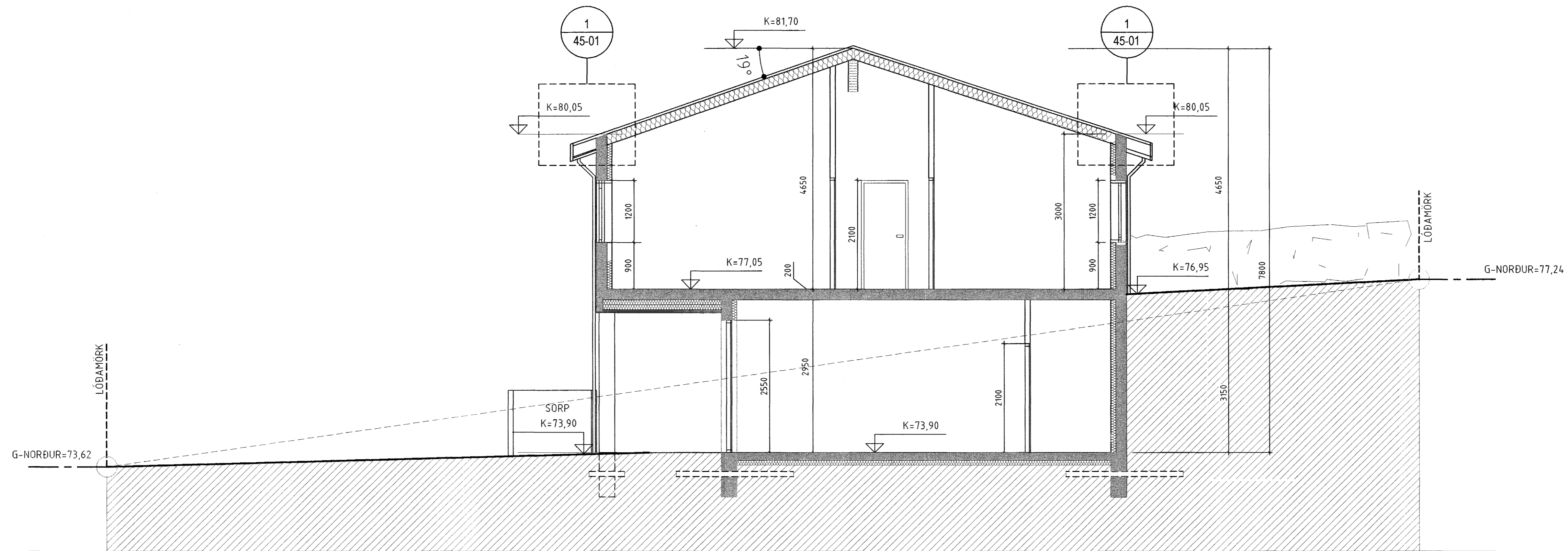
SNEIÐING A-A 1:50
