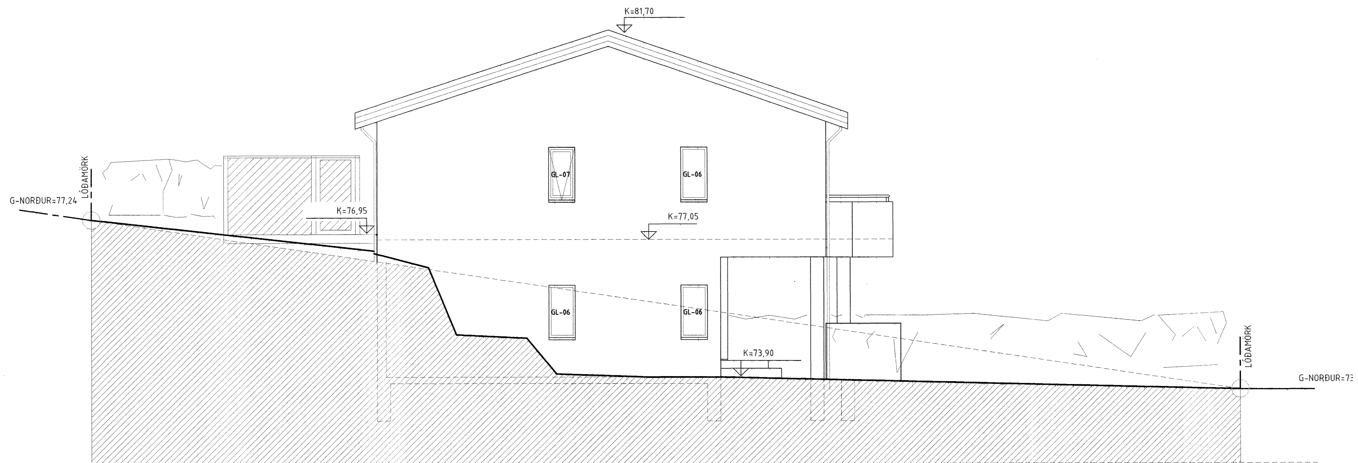
ÚTLIT SUÐUR 1:50
