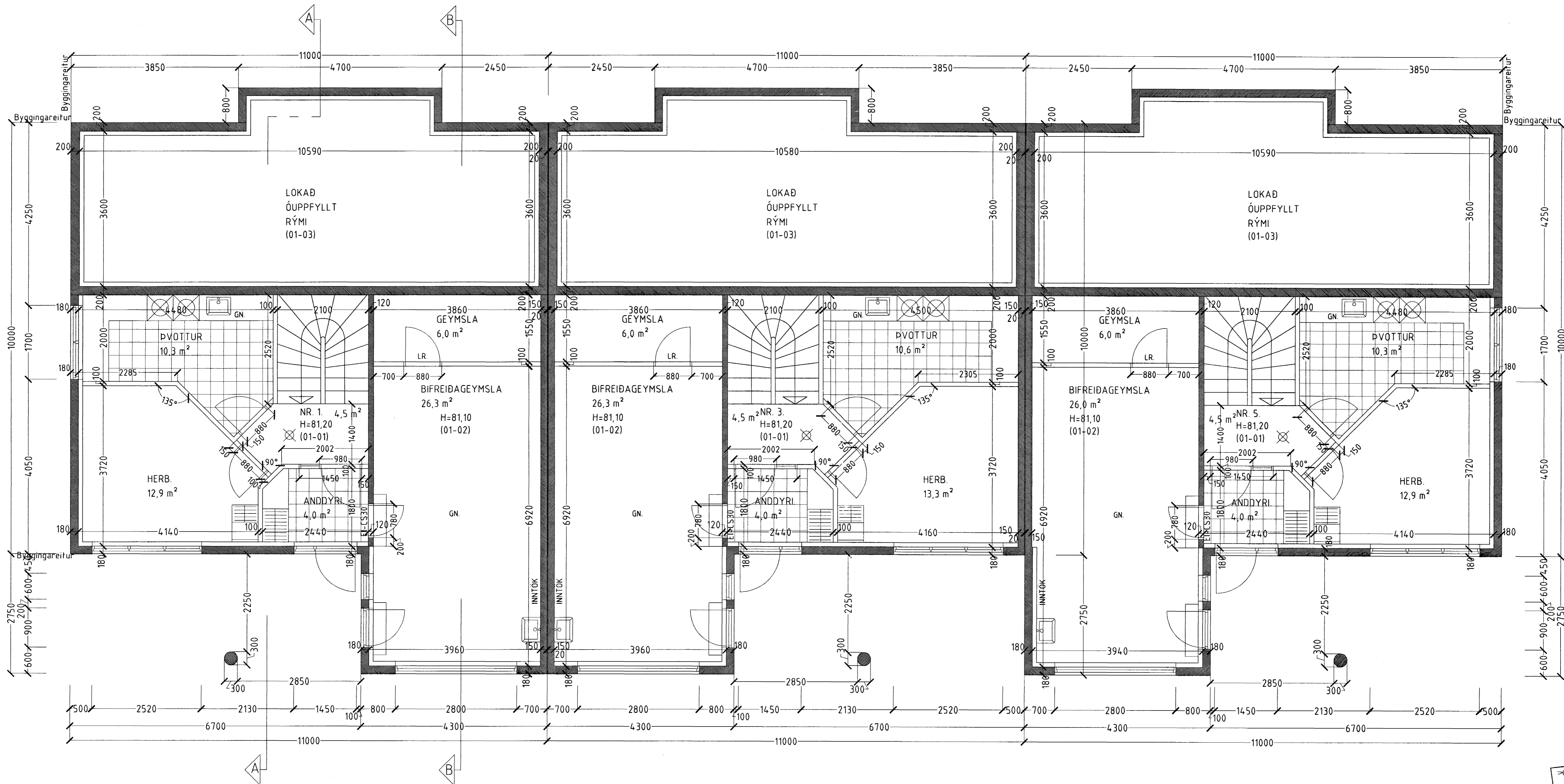
GRUNNMYND 1 HÆÐ. M. 1:50.
