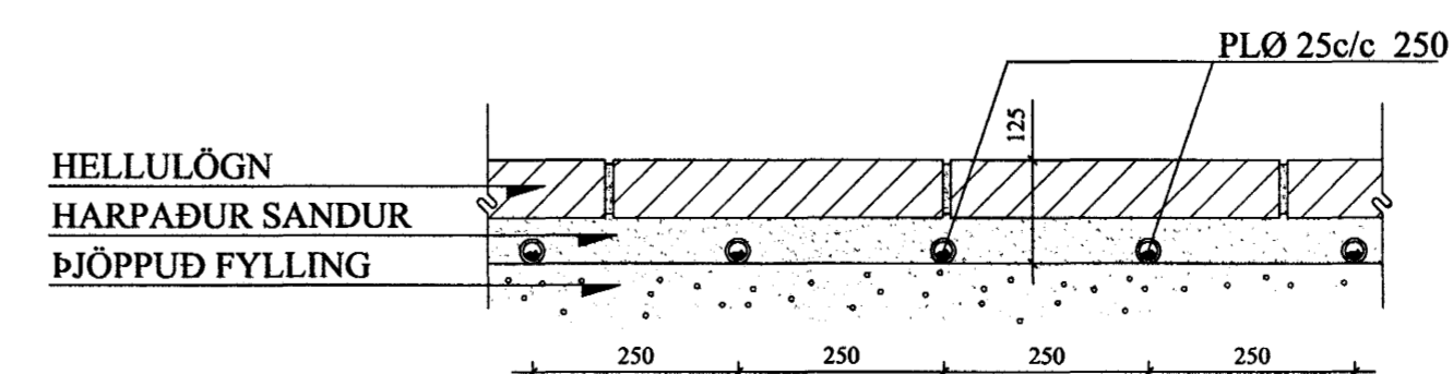
SNIÐ X - X. 1:10
