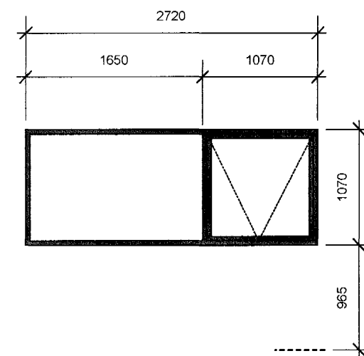
G17 HERBERGI 2.H KARMAR: 50X124 1 STK
