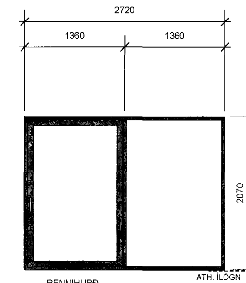
H3 BORÐSTOFA 1.H GLUGGI MED RENNIIHURÐ SEM OPNAST ÚT TIL HLIÐAR KARMAR: 50X124 1 STK
