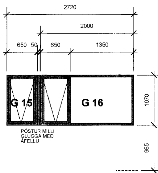
G15 BADHERB. 2.H EINN FRISTANDANDI, EINN EINS OG Á MYND MED PÓST Á MILLI GLUGGA MED ÁFELLU KARMAR: 50X124 2 STK
