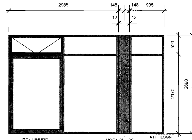
H2 STOFA GLUGGI MED RENNIIHURÐ SEM OPNAST ÚT TIL HLIÐAR HORNSTYKKI KLÆTT MED ÁFELLU KARMAR: 50X149 1 STK
