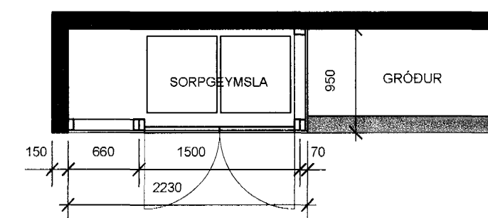
H6 SORPGEYMSLA TRÉKARMAR OG HURÐIR HURÐIR KLÆDDAR MED SAMSV. KLÆDNINGU OG Á HÚSI KARMAR: 50X115 1 STK
