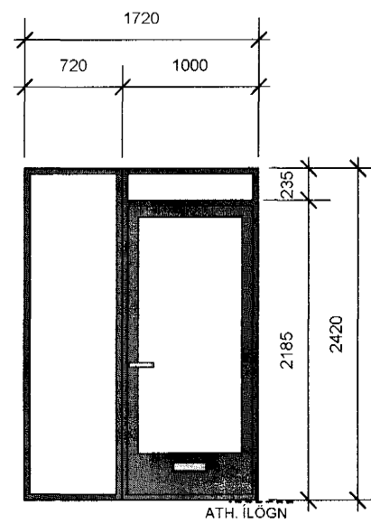
H1 ANDDYRI 1.H BRÉFALÜGA ÚR STÁLI KARMAR: 50X124 OPNAST INN 1 STK
