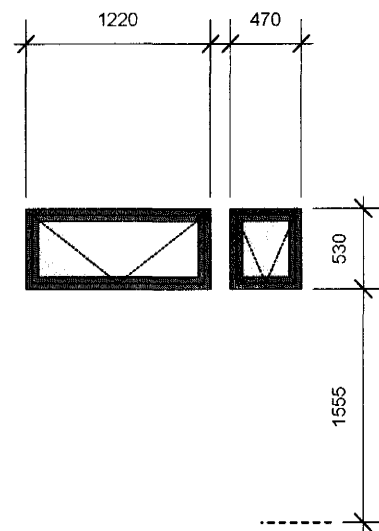
G6 ÞVOTTAHÚS 1.H SANDBLÁSÍÐ GLER KARMAR: 50X124 1 STK
