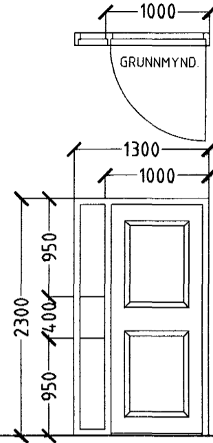
1 STK. ANDDYRI. HURÐ OPNAST HÆGRI ÚT.
