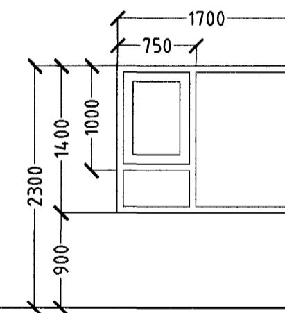
2 STK. HERB./HJÓN. BJÖRGUNAROP
