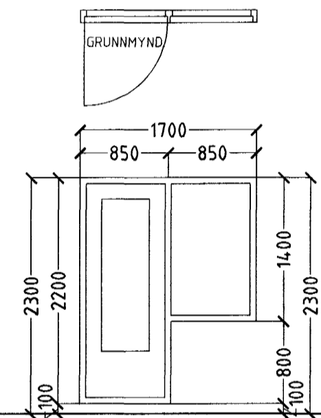
1 STK. STOFA/ELDHÚS. HURÐ OPNAST VINSTRI ÚT.
