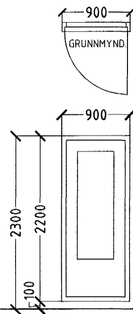
1 STK. STOFA. HURÐ OPNAST HÆGRI ÚT.
