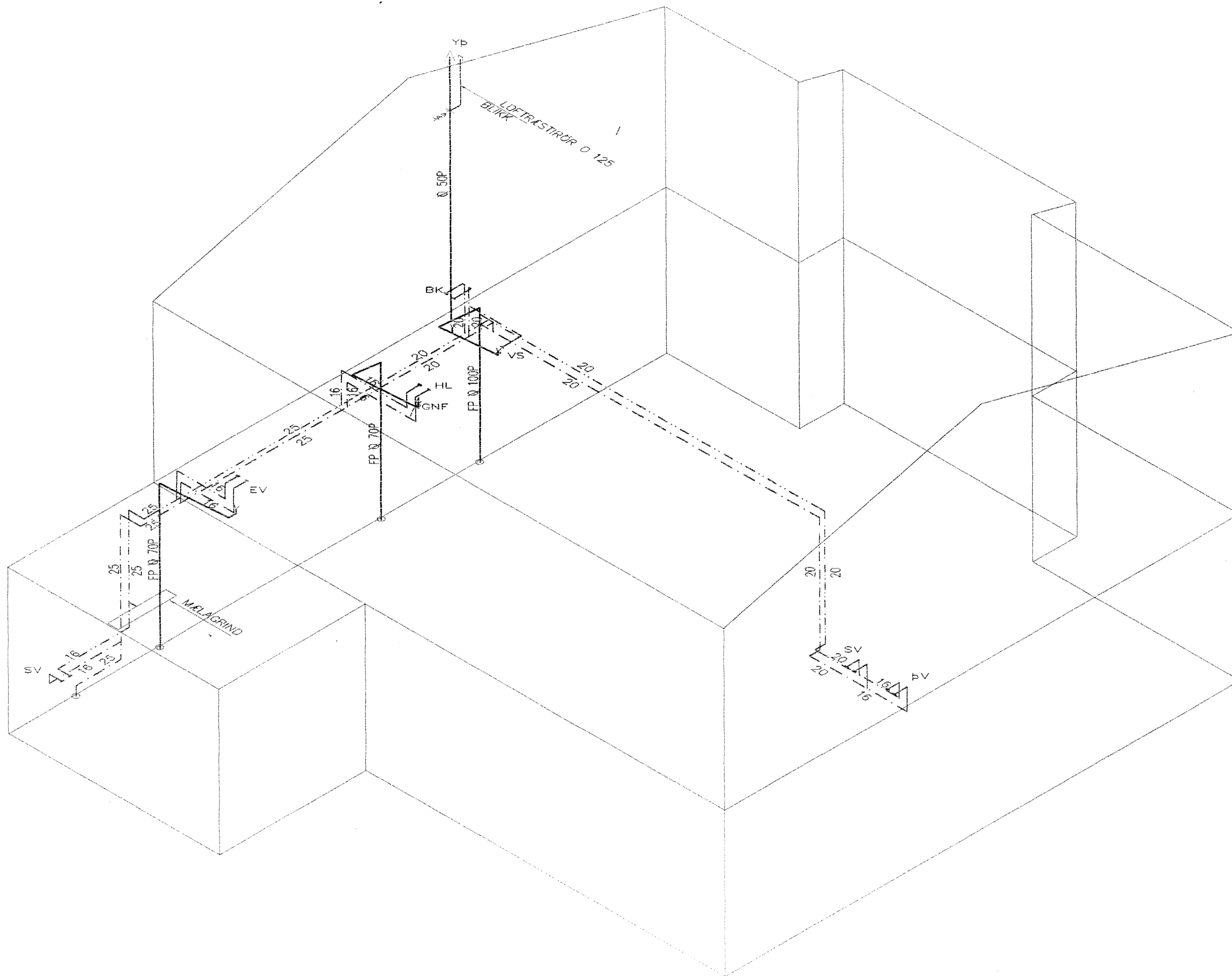
RÖMMYND VATNS OG FRÁRENNSLISLAGNA 1:50
