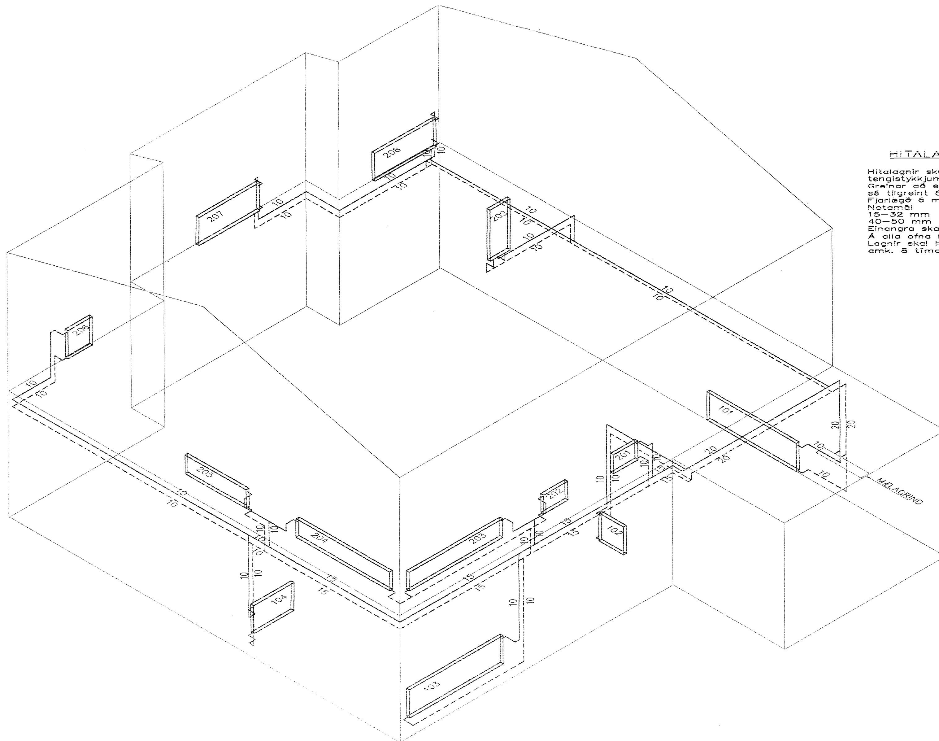
RÜMMYND HITALAGNA 1:50
