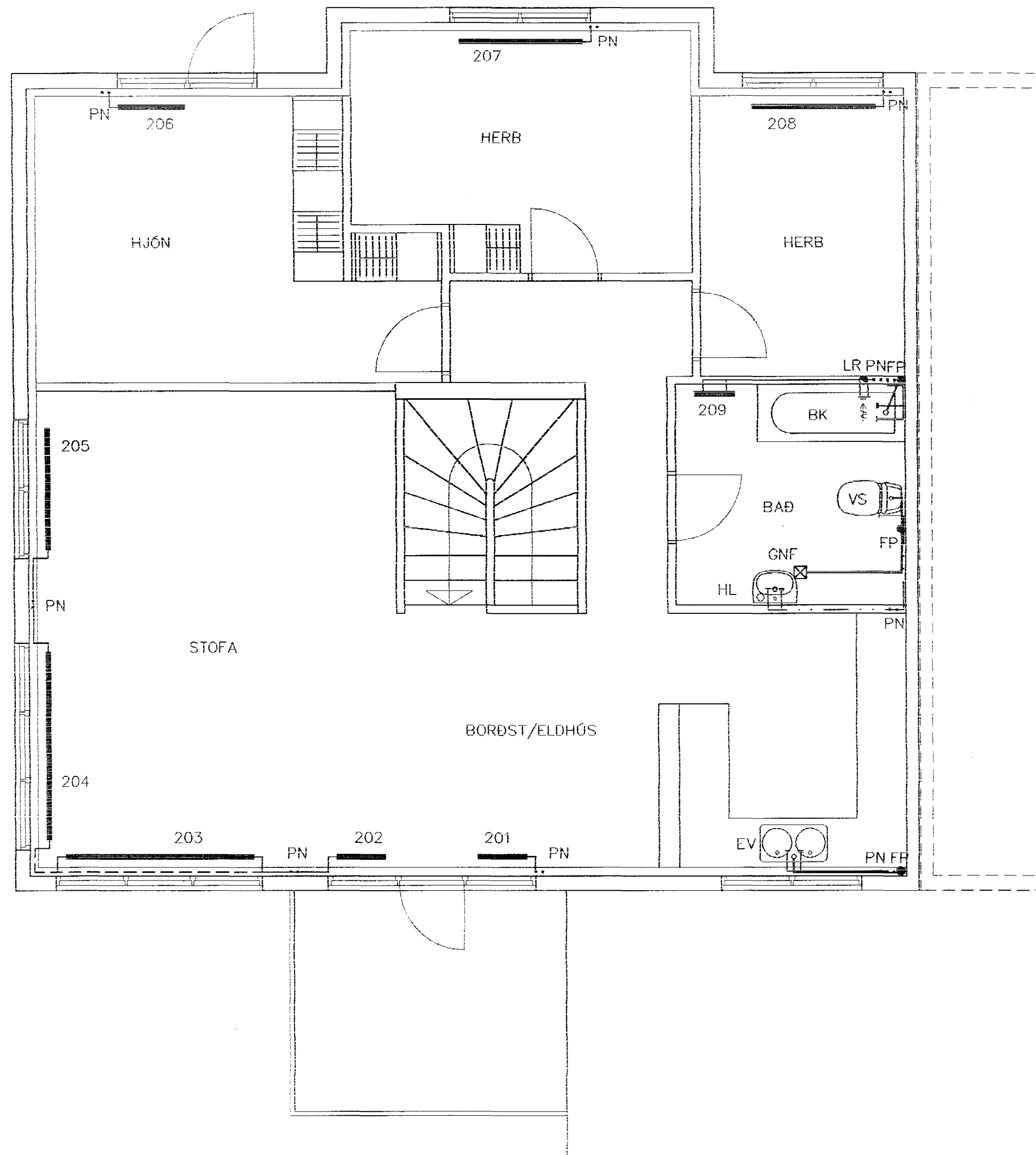
GRUNNMYND 2 HÆÐAR 1:50
