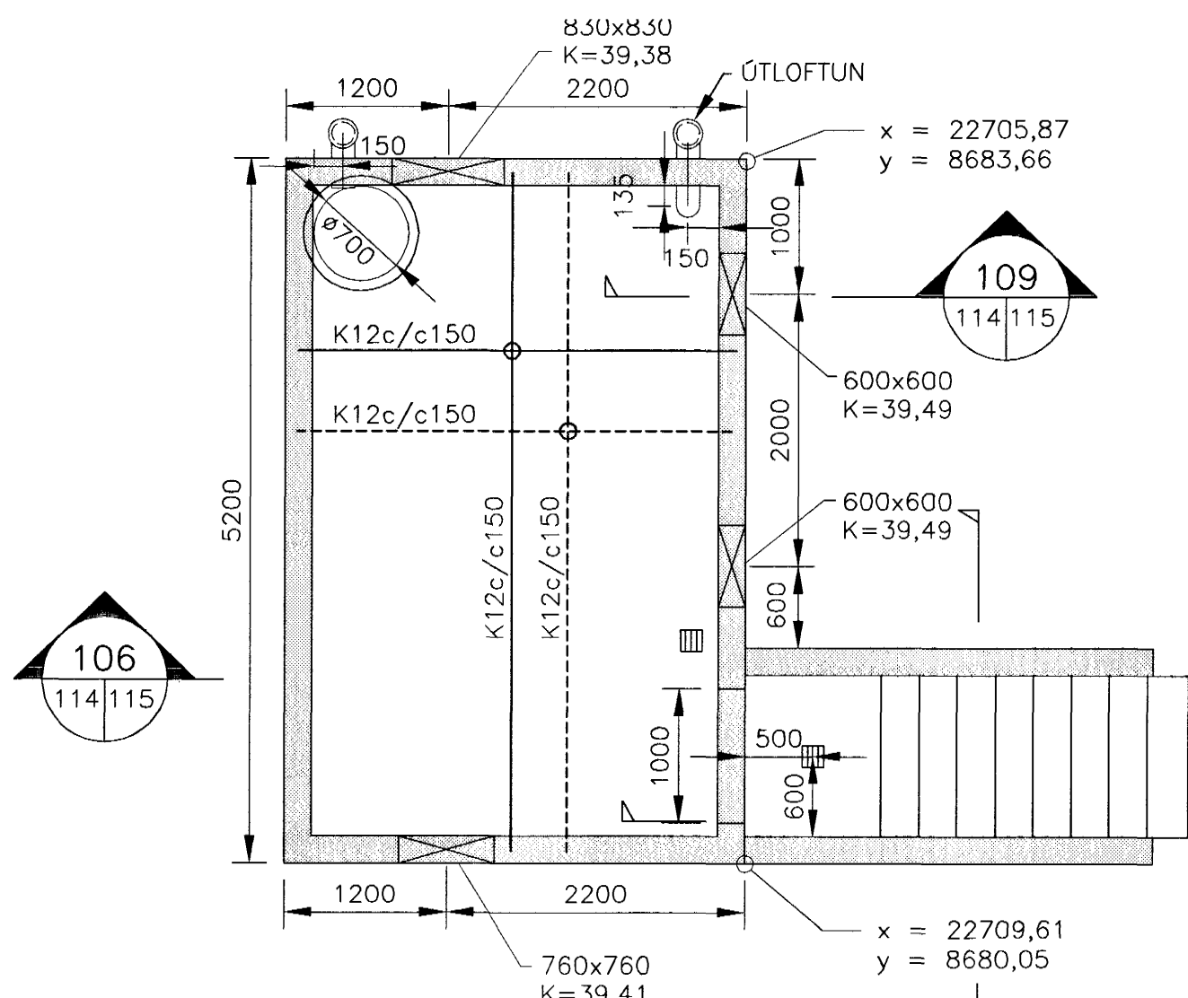
ÞAKPLATA GRUNNMYND, 1:50
