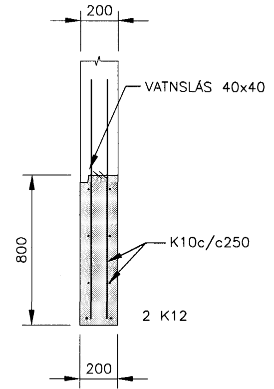
102 SNID 114|114 1:20
