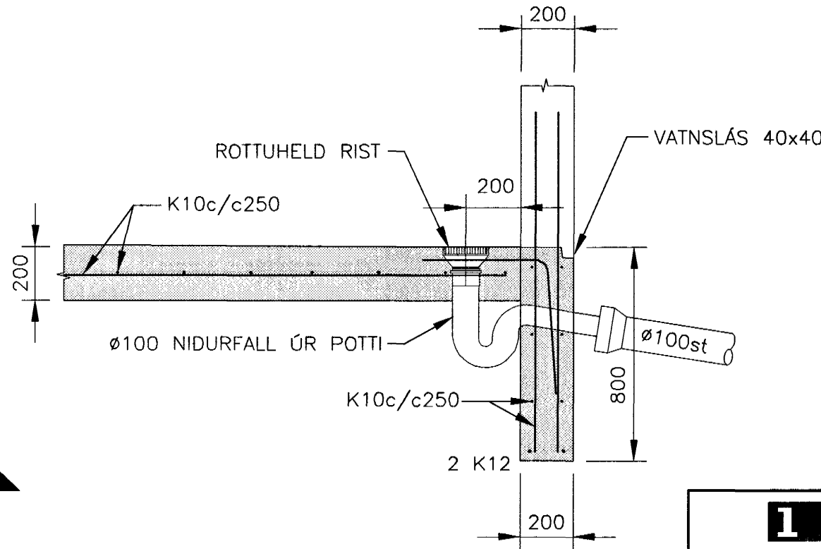
105 SNID 114|114 1:20
