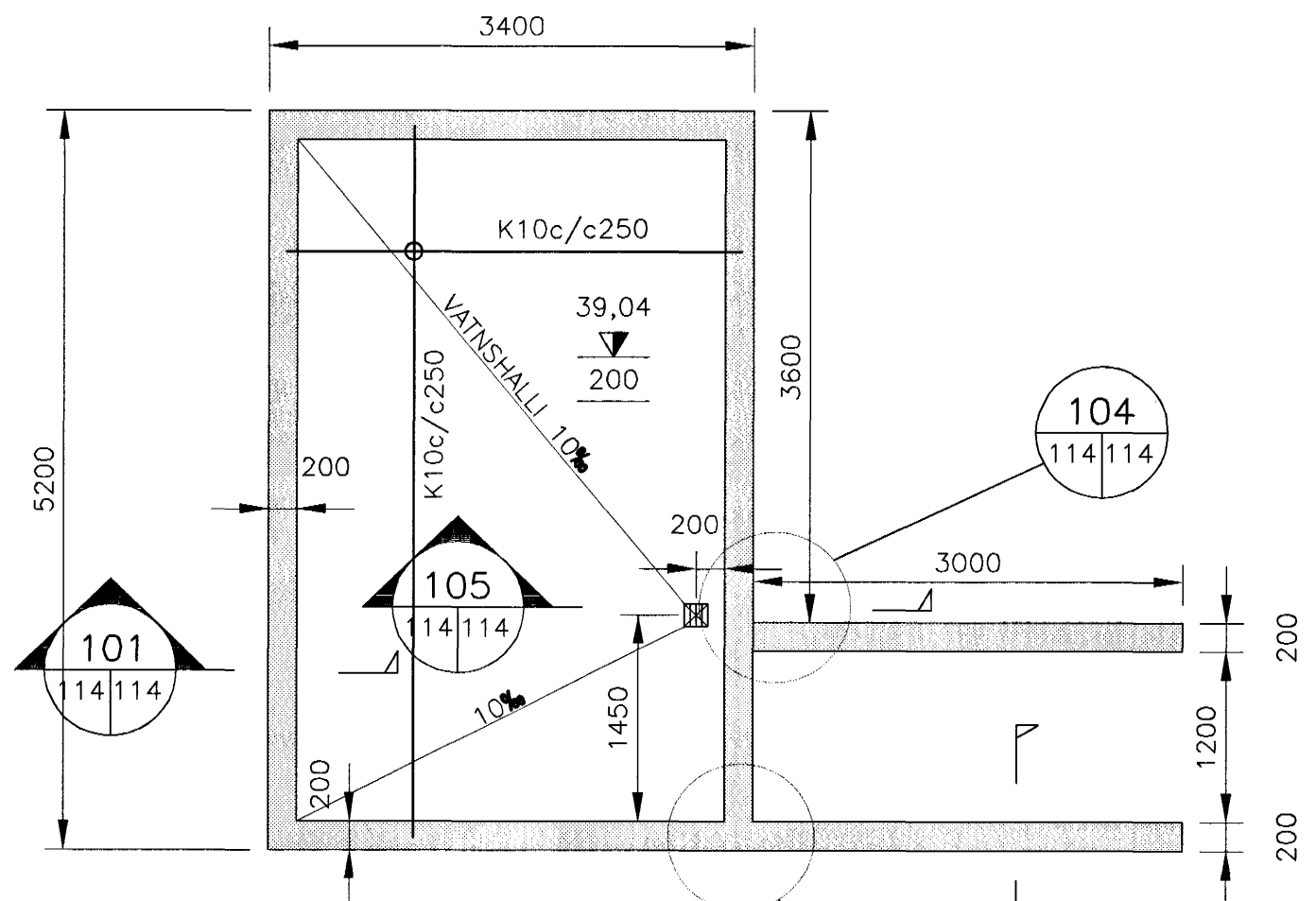
SÖKKLAR GRUNNMYND, 1:50
