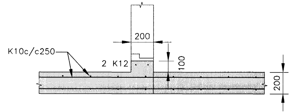
103 DEILI 114|114 1:20
