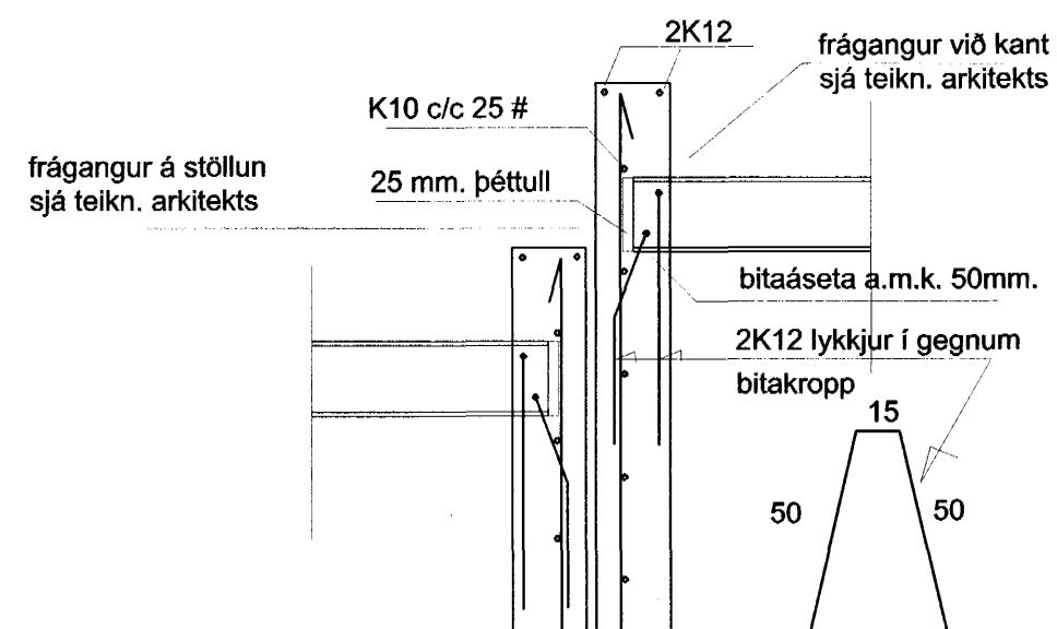
SNID D-D 1:20
