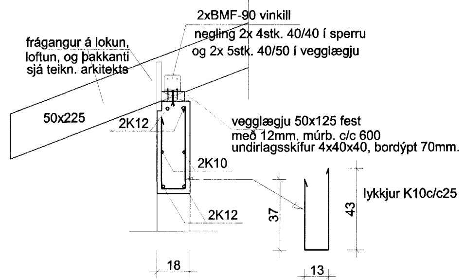
SNID A-A 1:20
