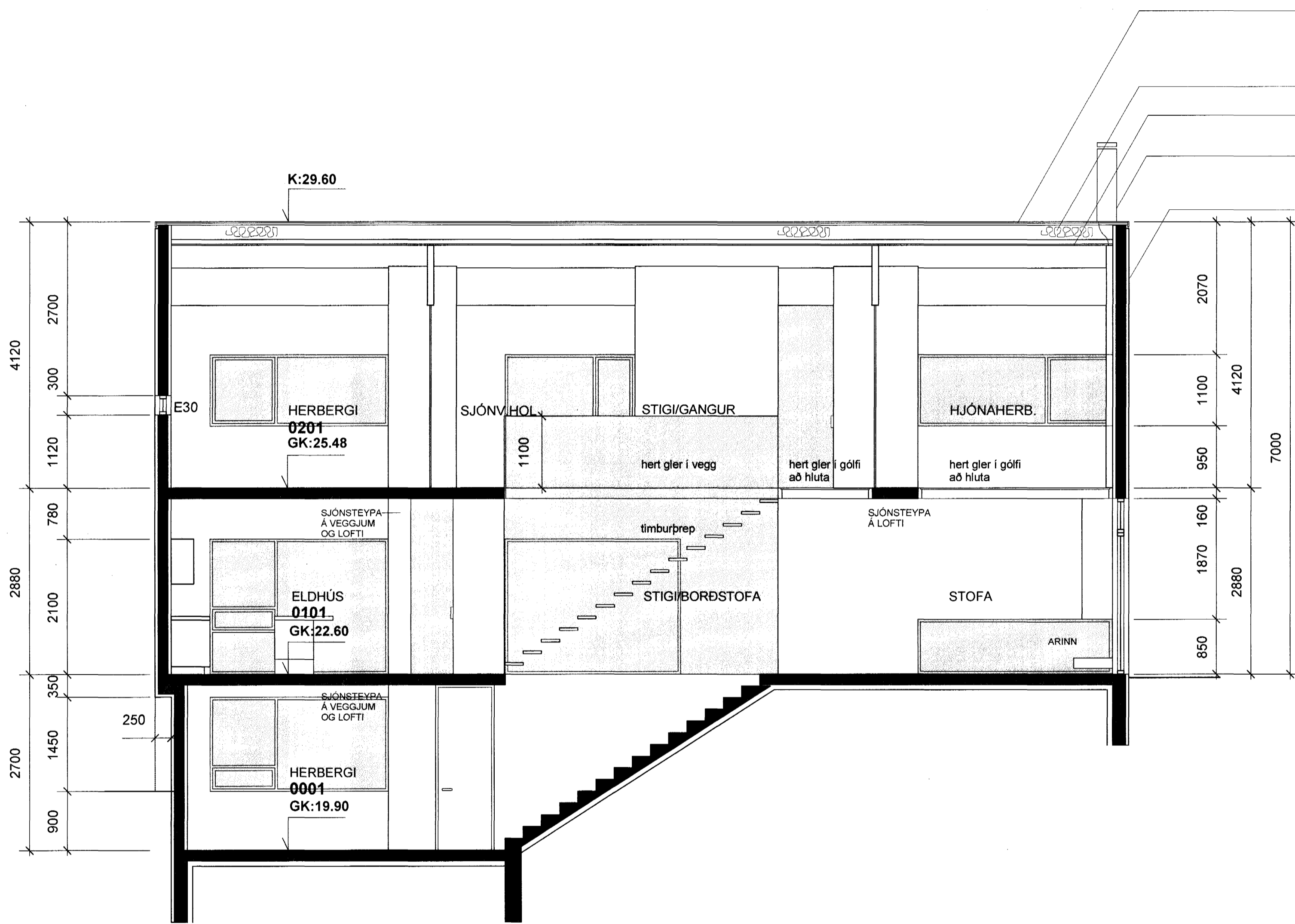
SNID A-A
