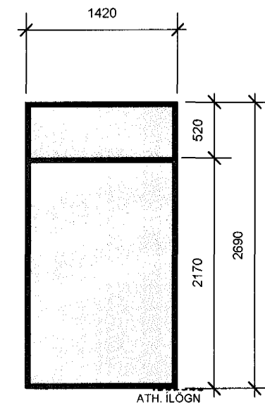
G3 STOFA 1.H KARMAR: 50X149 1 STK
