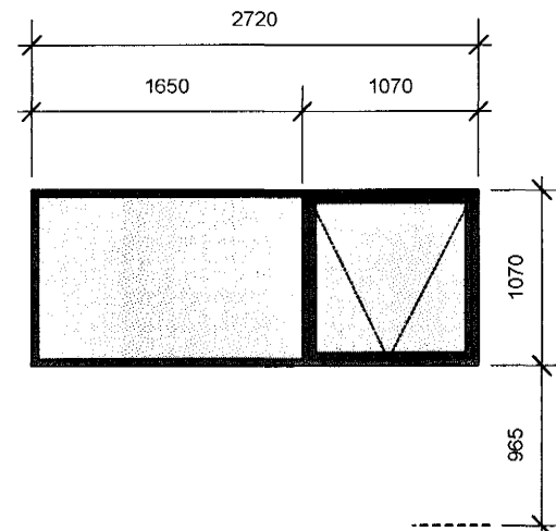
G18 HERBERGI 2.H KARMAR: 50X124 1 STK
