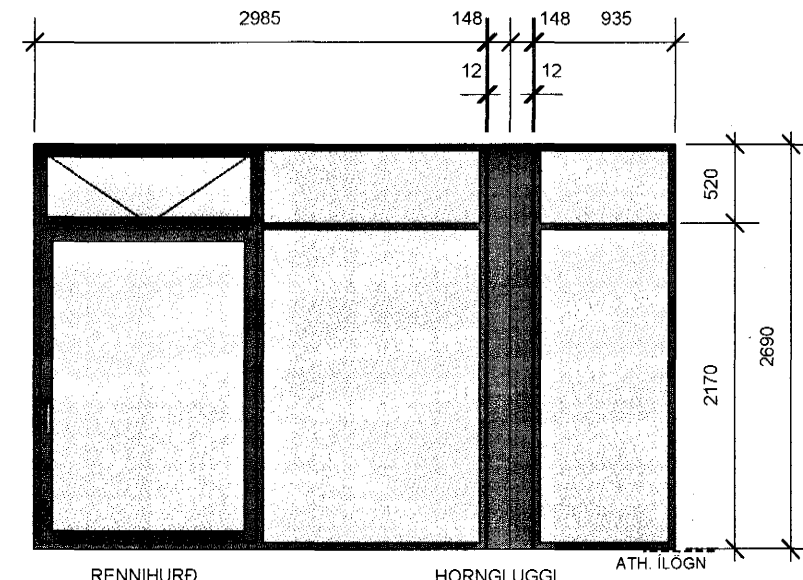
H2 STOFA GLUGGI MÆÐ RENNIHURÐ SEM OPNAST ÚT TIL HLIÐAR HORNSTYKKI KLÆTT MÆÐ AFÉLLU KARMAR: 50X149 1 STK
