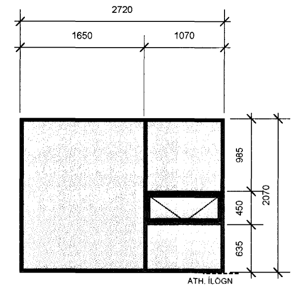
G5 ELDHÚS 1.H KARMAR: 50X124 1 STK
