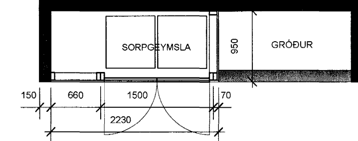
SORPGEYMSLA TRÉKARMAR OG HURDIR HURDIR KLÆDDAR MÆÐ SAMSV. KLÆÐNINGU OG Á HÚSI. KARMAR: 50X115 1 STK
