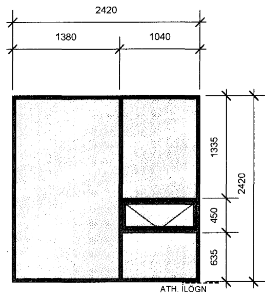
G1 HERBERGI 1.H KARMAR: 50X124 1 STK
