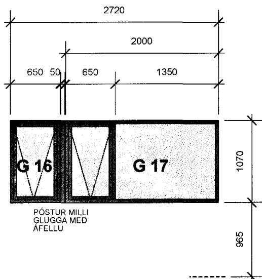
G16 BADHERB 2.H EINN FRÍSTANDANDI, EINN EINS OG Á MYND MÆÐ POST Á MILLI GLUGGA MÆÐ AFÉLLU KARMAR: 50X124 2 STK
