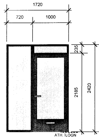
H1 ANDDYRI 1.H BRÉFALUGA ÚR STÁLI KARMAR: 50X124 OPNAST INN 1 STK
