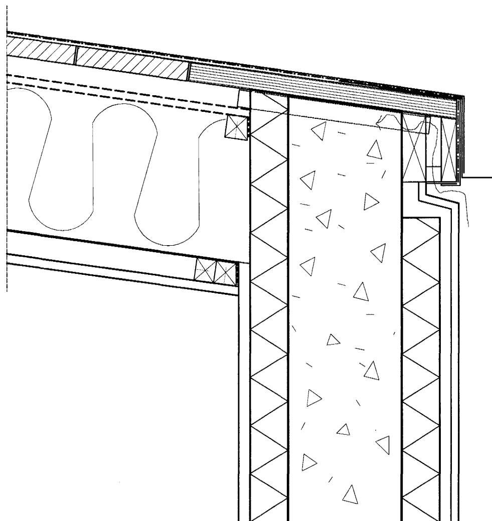
402 LÓÐRÉTT SNIÐ EINHALLA ÞAK; LANGHLIÐ
