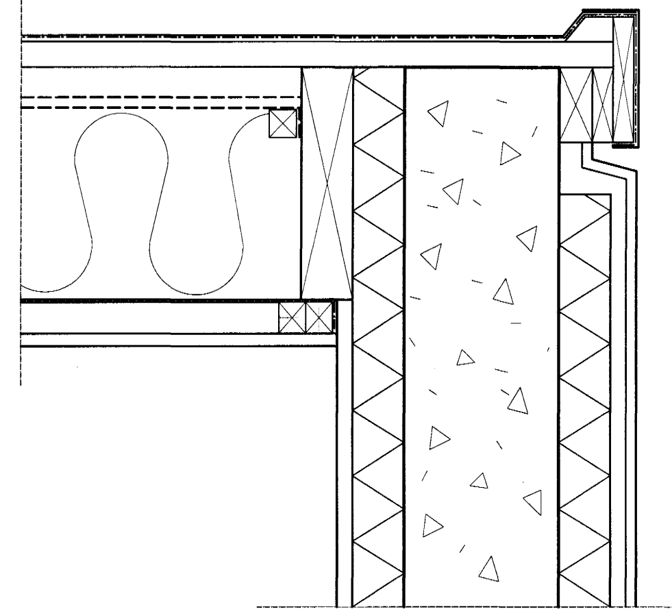
403 LÓÐRÉTT SNIÐ EINHALLA ÞAK; GAFLAR
