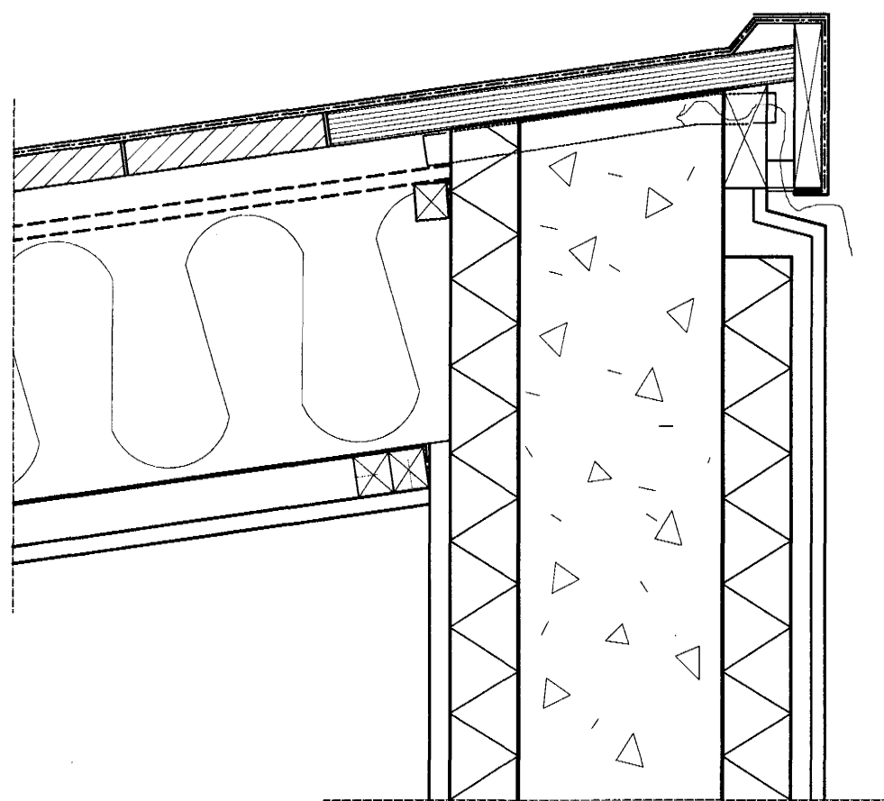
401 LÓÐRÉTT SNIÐ EINHALLA ÞAK; LANGHLIÐ
