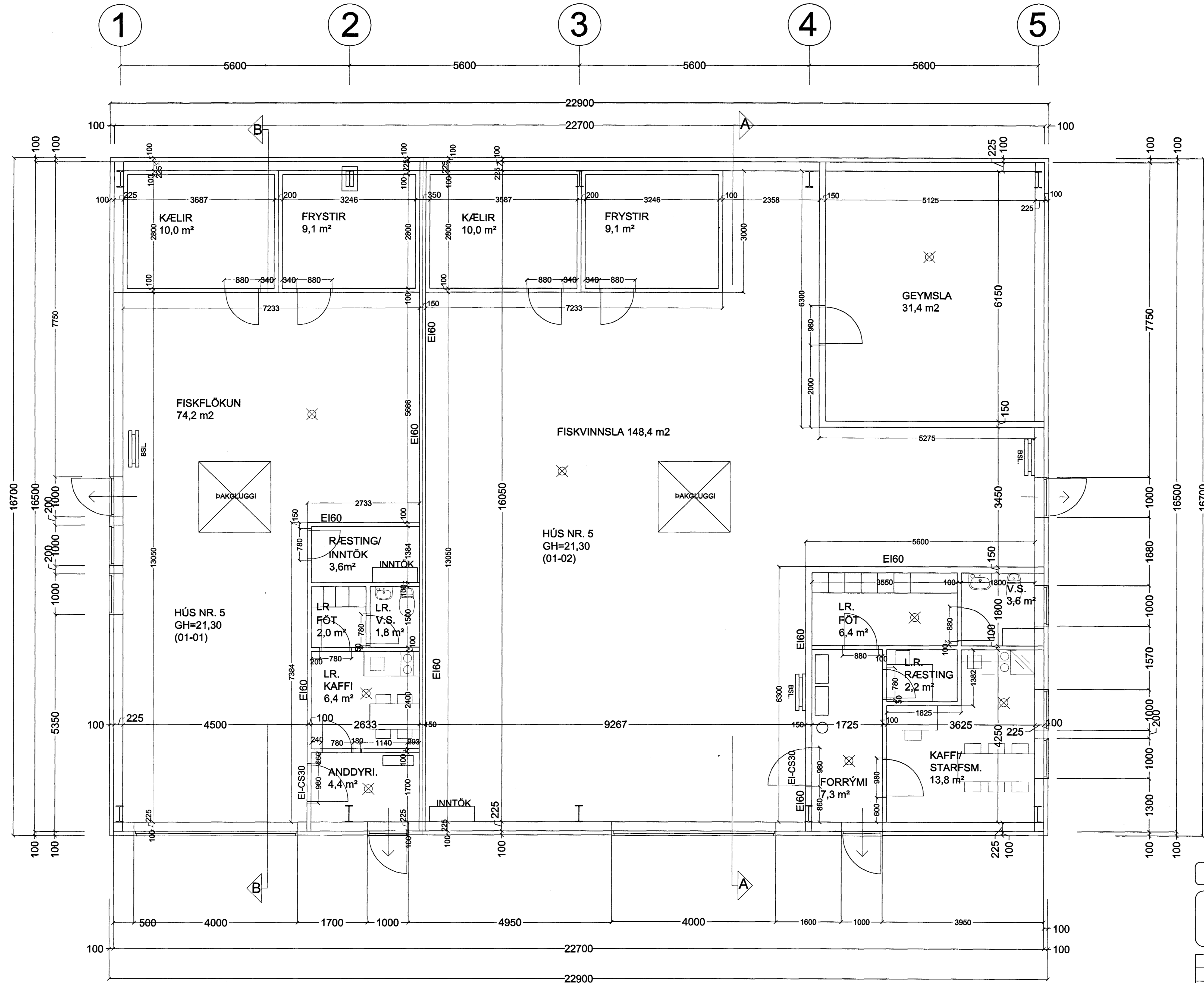
GRUNNMYND 1. HÆÐ MKV. 1:50.
