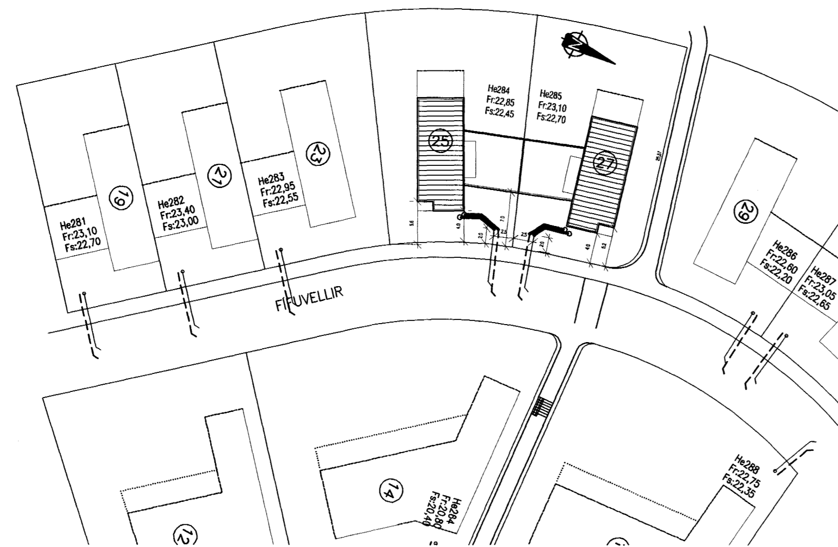
AFSTÖÐUMYND mkv. 1:500
