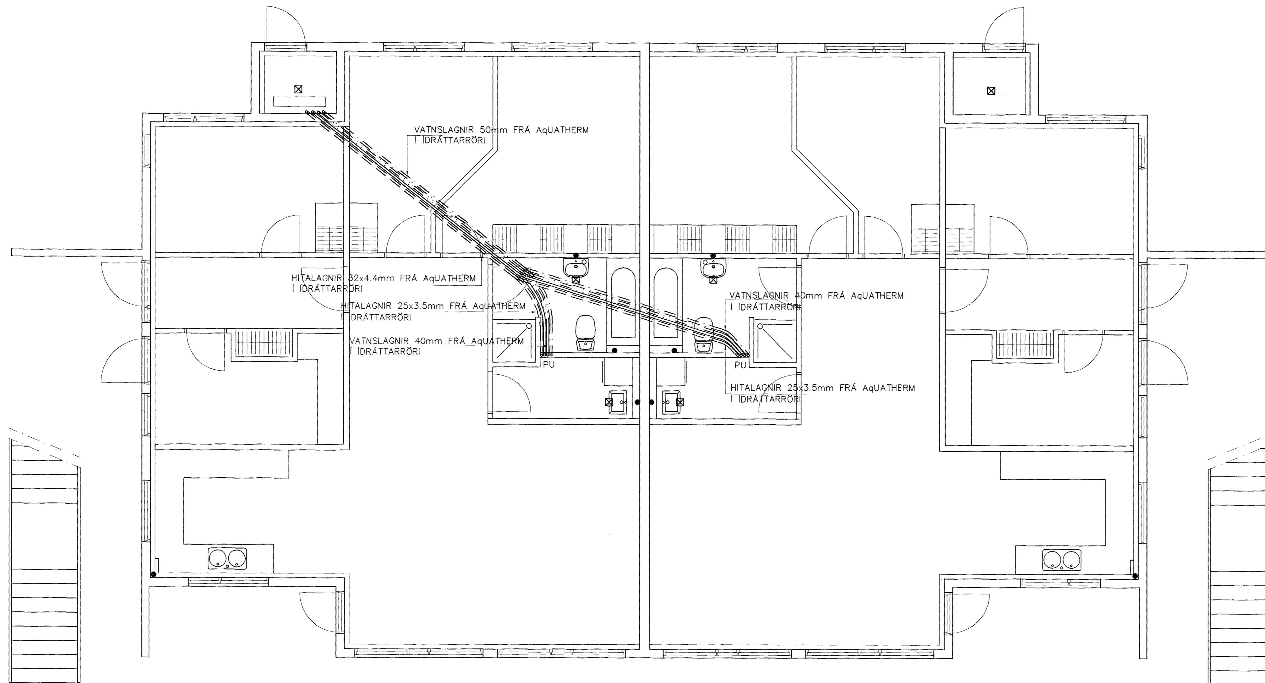
GRUNNMYND 1: 50
